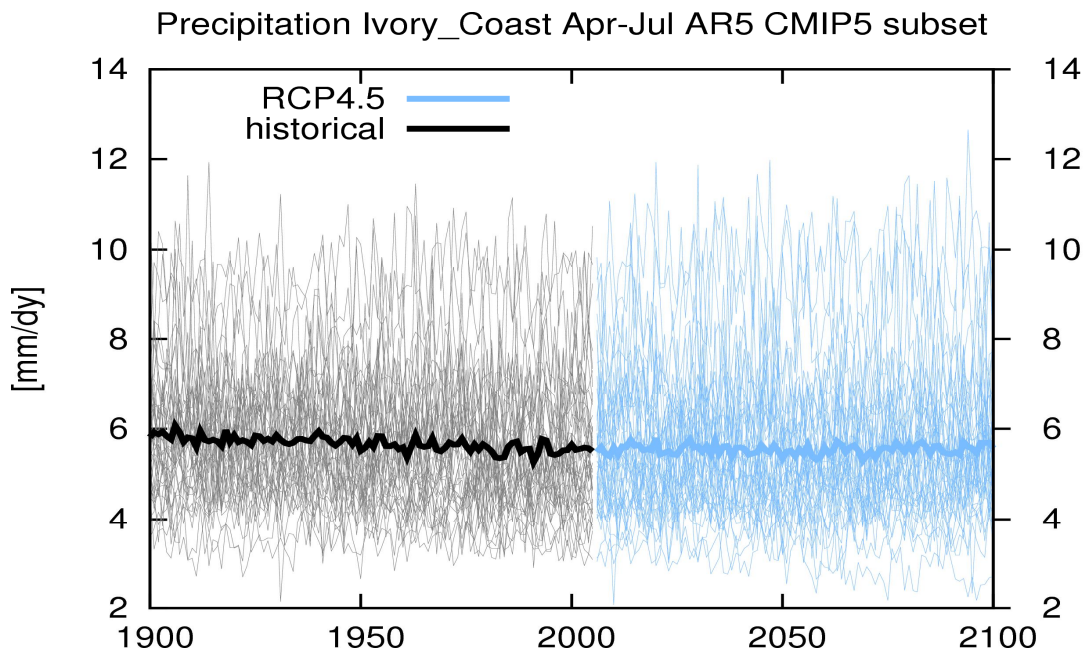
Figure8 : Scénario évolution de la pluviométrie journalière moyenne de 2000 à 2100
