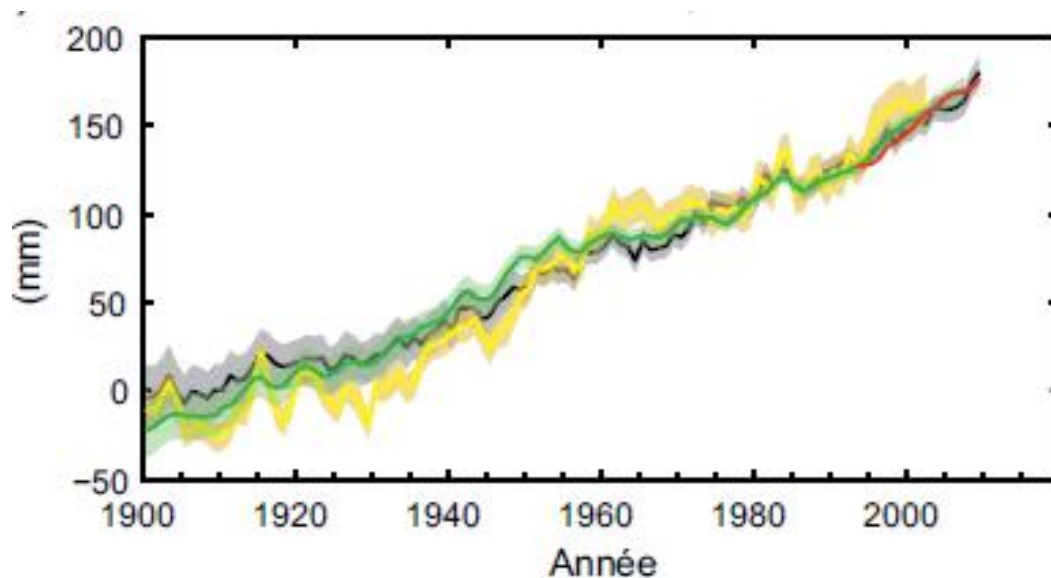
Figure 3 : Évolution du niveau moyen des mers (GIEC, 2013)
