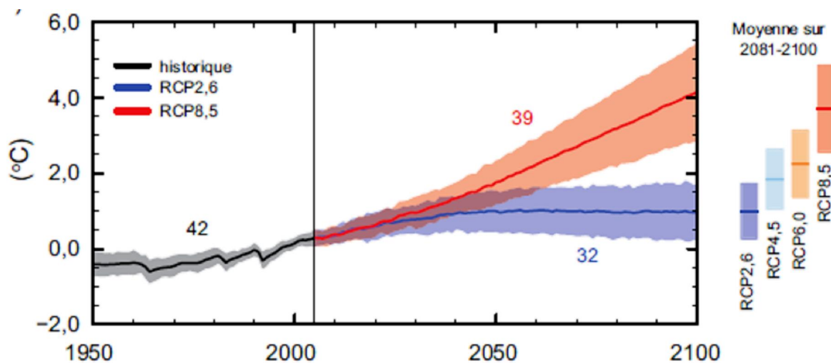
Figure 5 : Évolution de la température moyenne à la surface du globe (GIEC , 2013)
