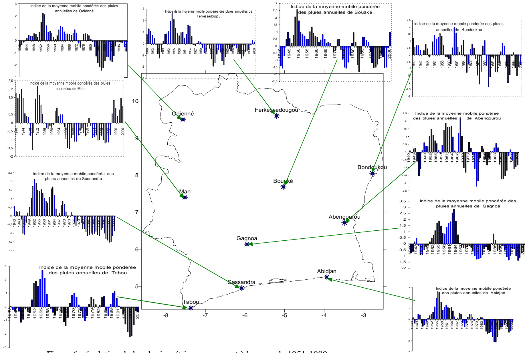
Figure 6 : évolution de la pluviométrie par rapport à la normale 1951-1980 (SODEXAM)
