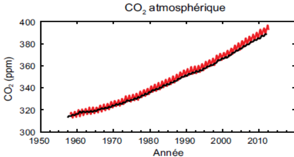
Figure 4 : Evolution du CO 2 atmosphérique (GIEC, 2013)
