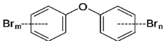
Figura 4. Struktura e polibrom difenil etereve (PBDEs)
