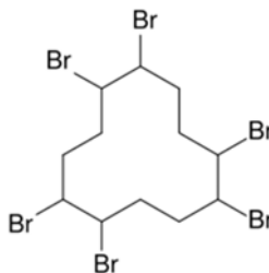
Figura 6. Formula strukturore e HBCD
