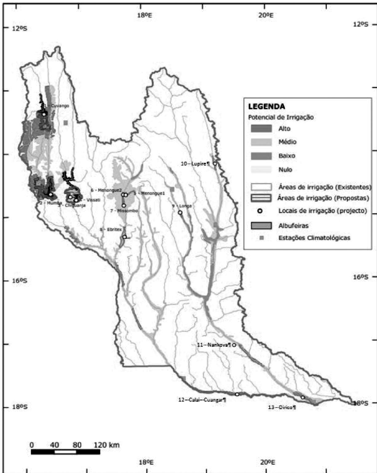
Figura 6.12 – Localização dos pontos de irrigação existentes e propostos
