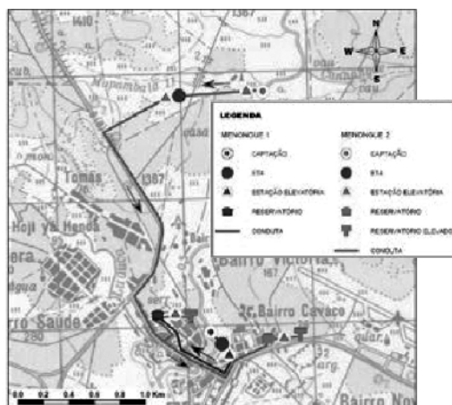
Figura 8.13 – Menongue. Esquema da solução base
