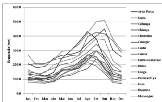
Figura 3.17 – Evaporação mensal média (1943-74)
