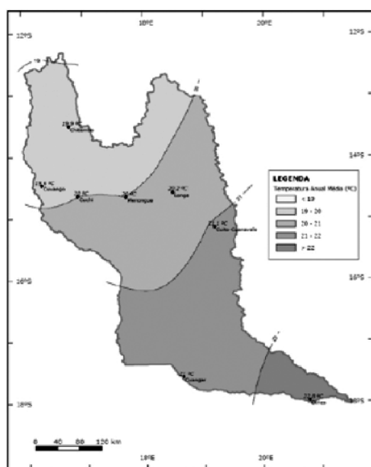
Figura 3.16 – Temperatura anual média
