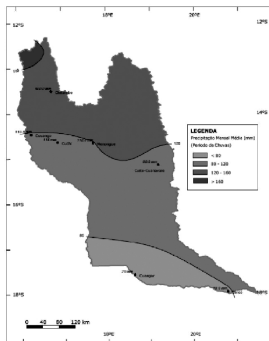
Figura 3.18 - Precipitação mensal média na época das chuvas (Outubro a Maio) (mm). Período de 1943 a 1974
