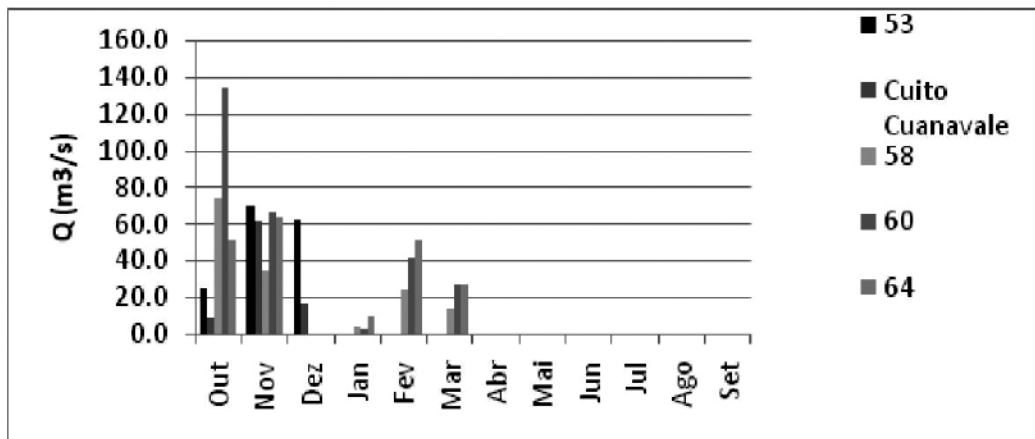
Figura 8.12 - Variação de caudal ecológico mensal médio durante o ano ao longo do rio Kuíto
