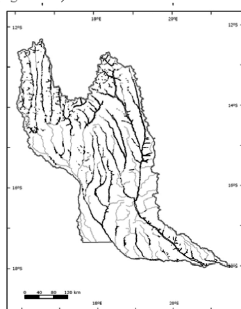
Figura 6.18 – Delimitação da área ocupada pelos leitos maiores de cheia
