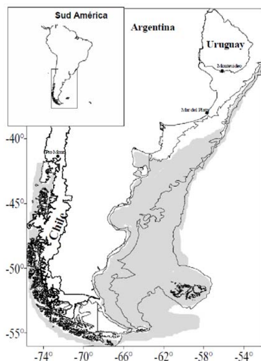
Figura 1. Distribución de Zygochlamys patagonica (en gris). Fuente: Bogazzi 2008.
