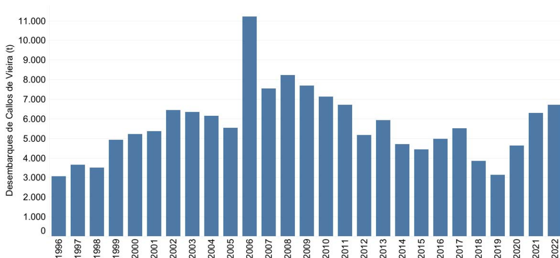
Figura 3. Desembarques anuales de callos de vieira (t). Fuente: Subsecretaría de Pesca y Acuicultura – SAGyP – MEC.
