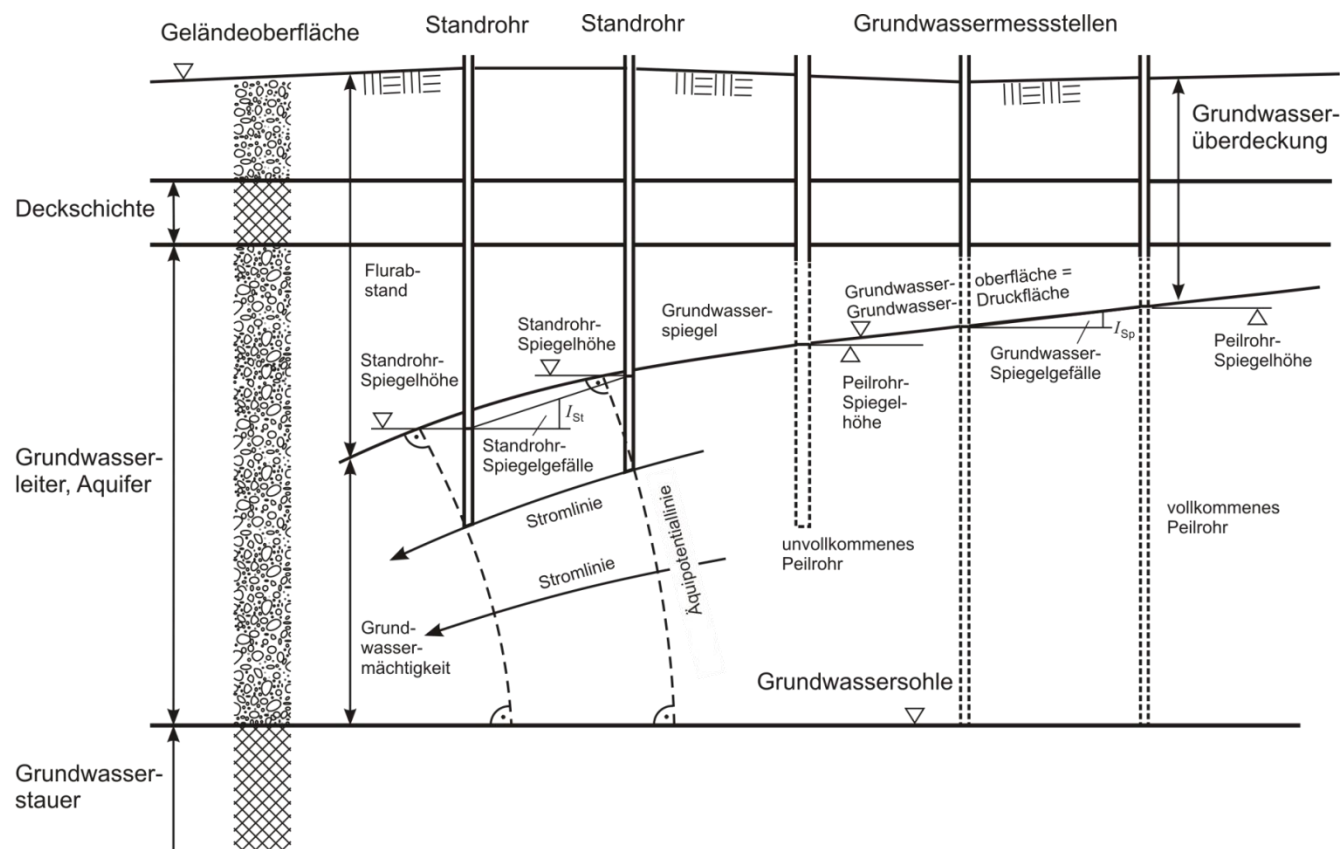
Bild B.2 — Freies Grundwasser – Vertikale Strömungsebene
