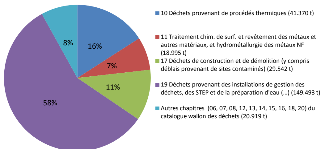
Figure 31 Exportation de déchets soumis à notification et consentement écrits préalables en 2014. Exportations depuis la Wallonie vers un pays tiers. Ventilation par chapitres du catalogue wallon des déchets. Source : DPD
