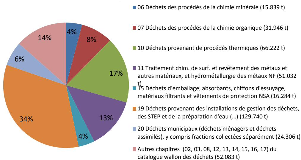
Figure 32 Importation de déchets soumis à notification et consentement écrits préalables en 2014. Importations vers la Wallonie depuis un pays tiers. Ventilation par chapitres du catalogue wallon des déchets. Source : DPD
