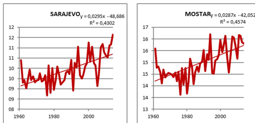
Slika 7: Trendovi promjena temperature zraka u Federaciji BiH, 1961–2016. (Sarajevo, Mostar) (Izvor: (Federalni hidrometeorološki zavod, FHMZ BiH)
