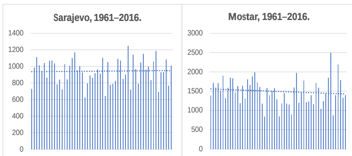
Slika 8: Trendovi promjena padavina u Federaciji BiH, 1961–2016. (Sarajevo, Mostar) (Izvor: Federalni hidrometeorološki zavod, FHMZ BiH)
