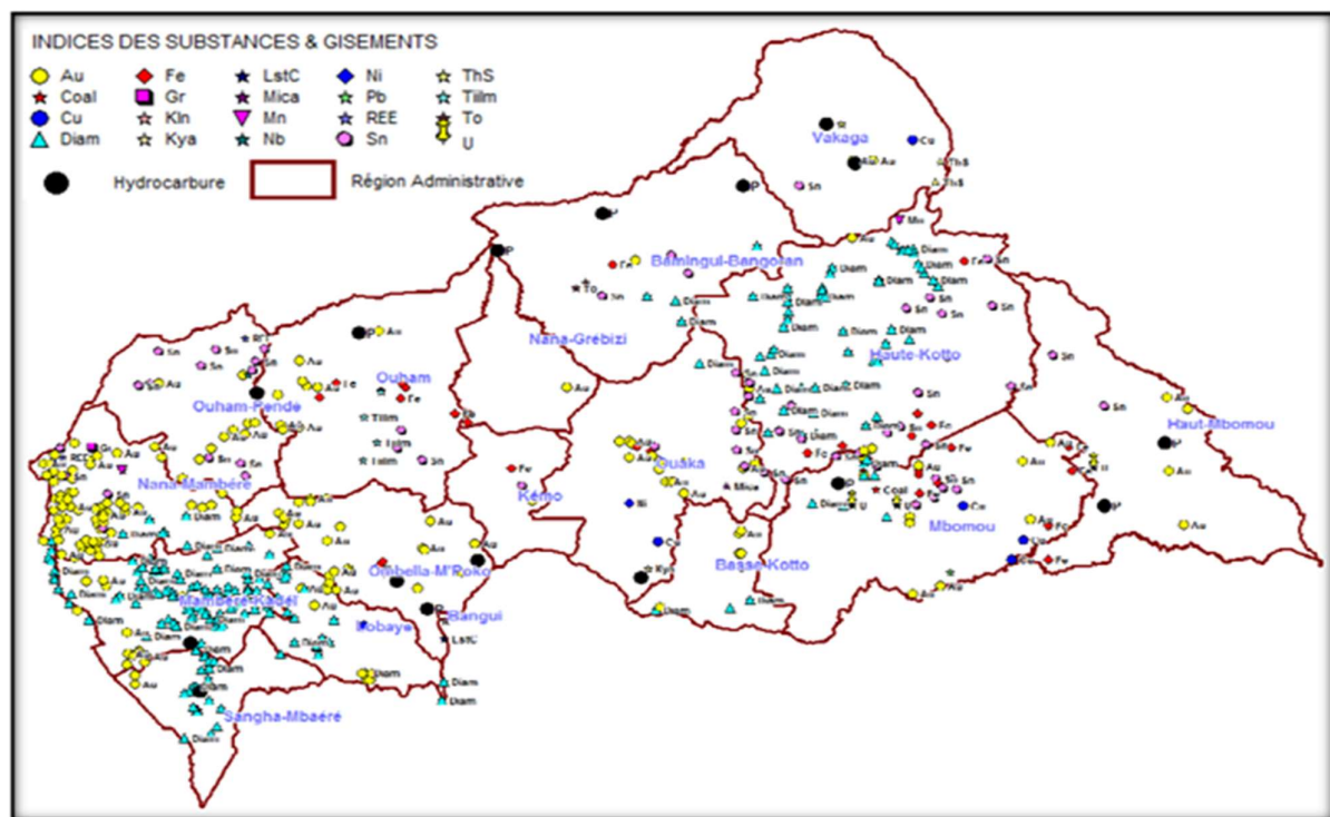
Figure 31 : Indices des substances & gisements (Géologie, Juillet 2017)
