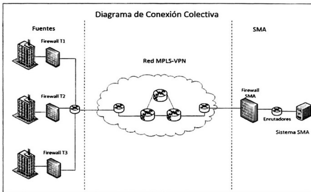
Figura 4: Diagrama de conexión Colectiva.
