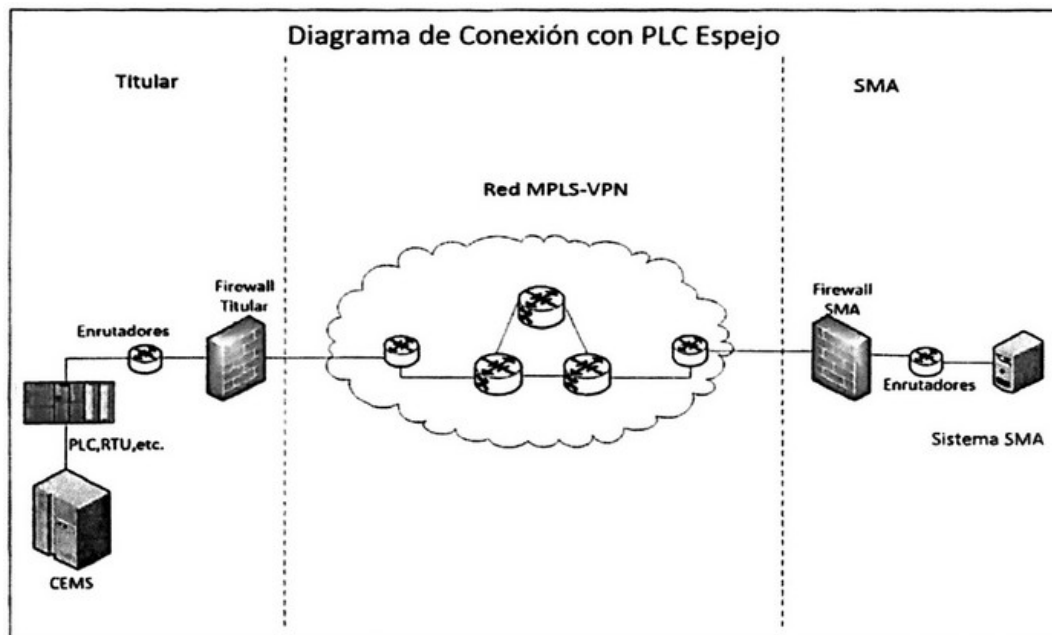
Figura 3: Diagrama de conexión con PLC Espejo
