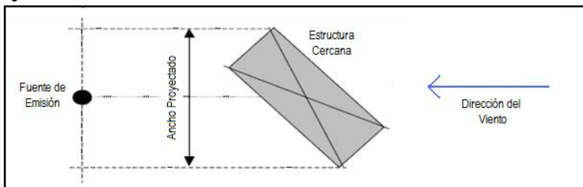
Figura 10. Determinación de la estructura cercana.
