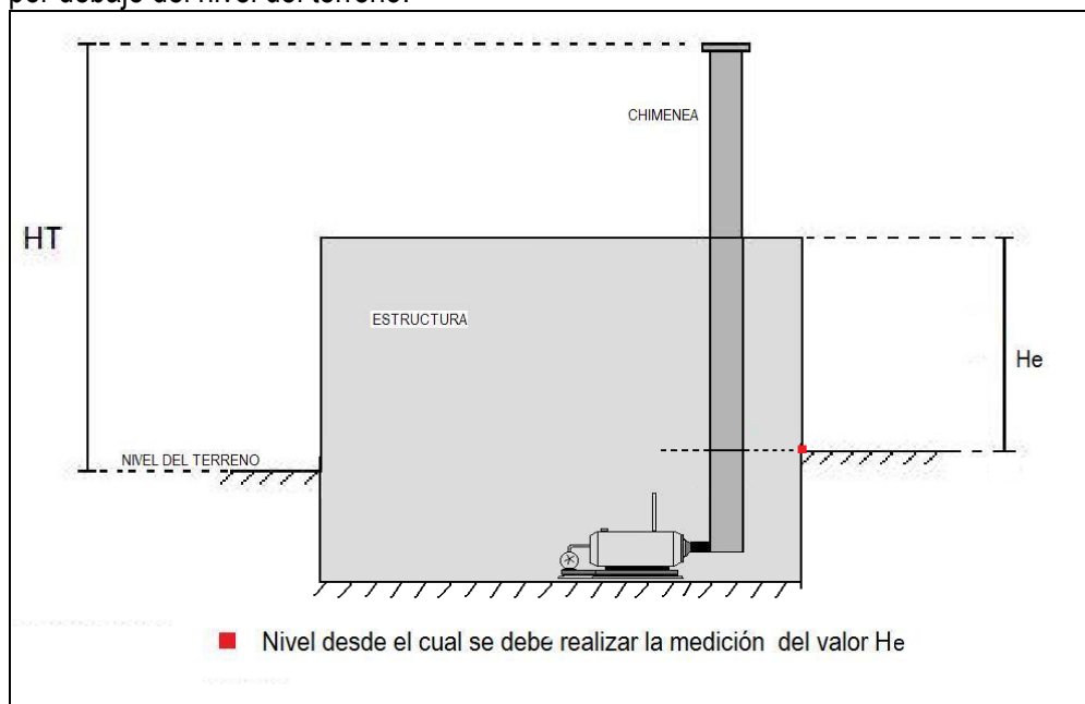
Figura 3. Determinación del valor H_e cuando el equipo o instalación que genera la emisión está por debajo del nivel del terreno.
