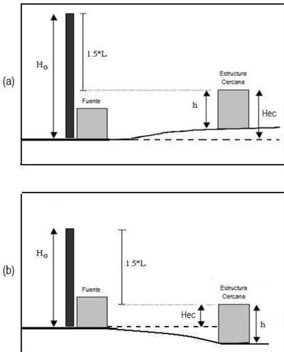
Figura 11. Determinación de las dimensiones de la estructura cercana
