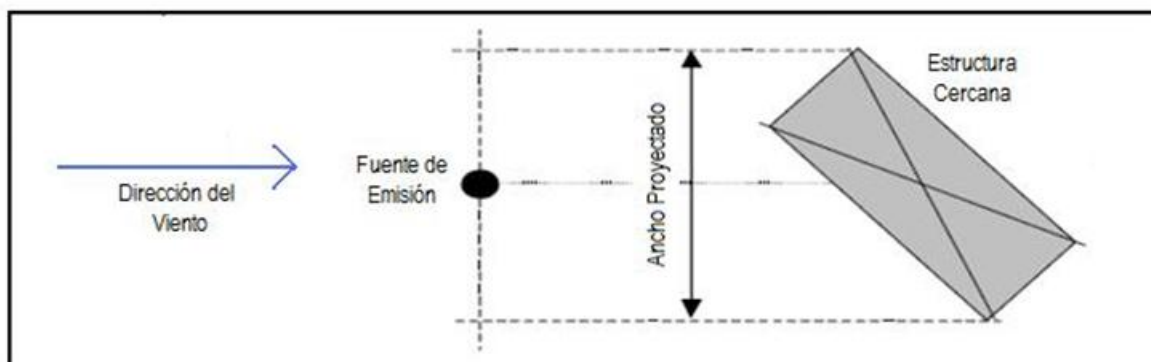
Figura 9. Determinación de la estructura cercana.
