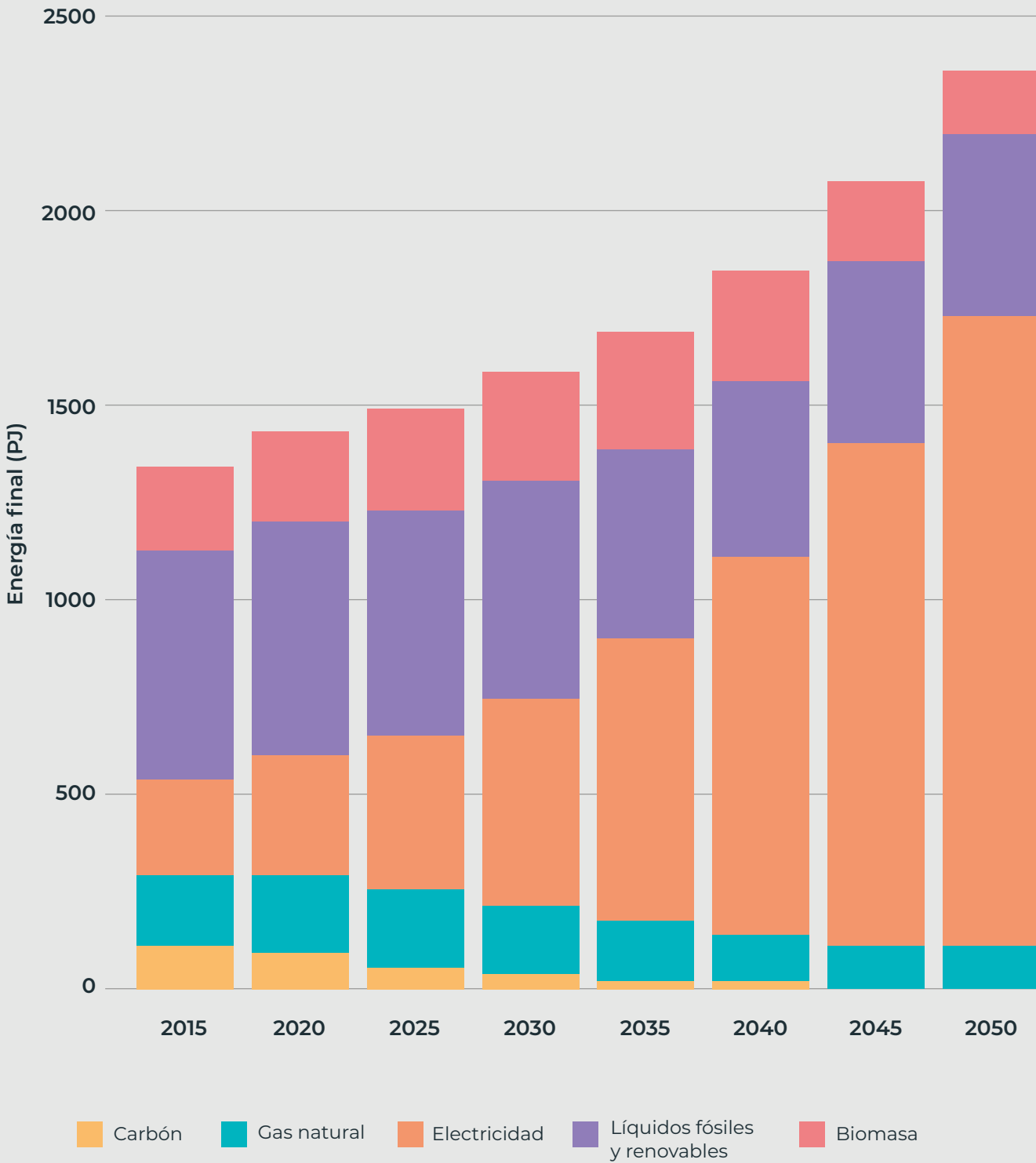
Figura 21. Composición de la generación eléctrica para alcanzar la carbono neutralidad en Colombia Fuente: E2050, Universidad de Los Andes et al. 2021; BID 2021.
