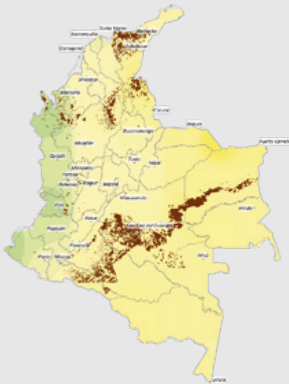
RCP 6.0
