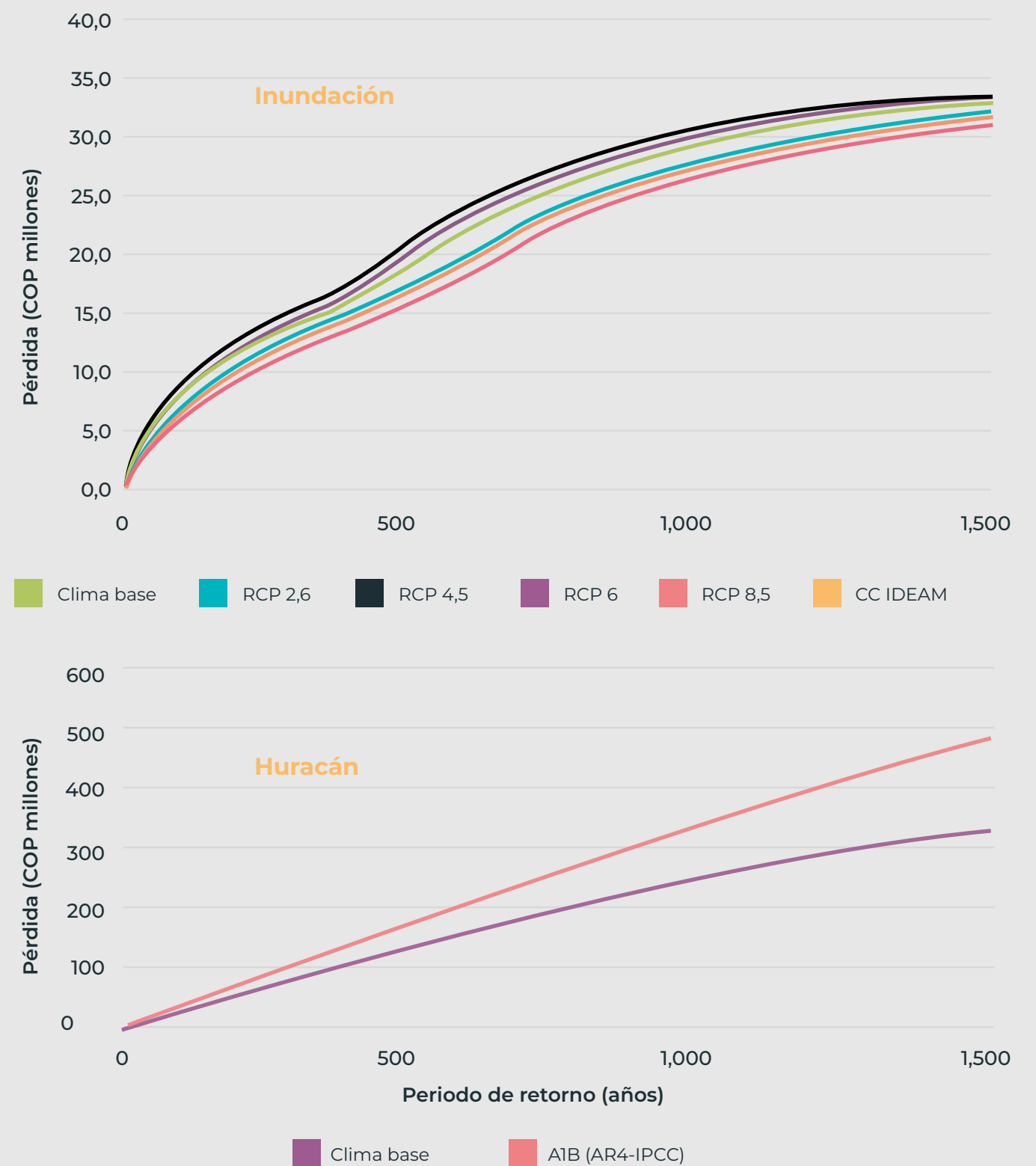
Figura 7. Curvas de pérdida máxima probable (PML) calculadas para todos los escenarios RCP y todas las amenazas climáticas consideradas (Ingeniar 2021)
