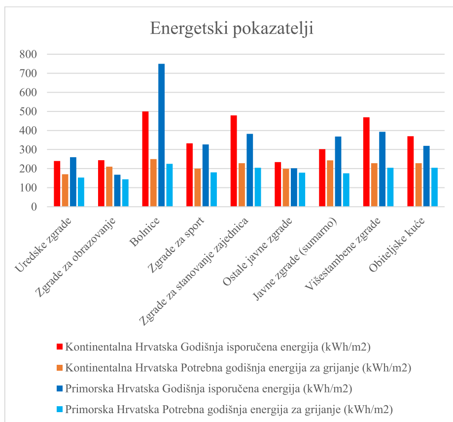
Slika 2.8 Energetski pokazatelji
