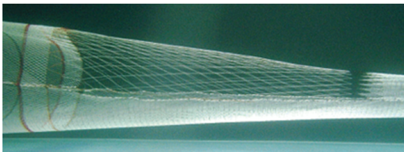
Fig. 2.1.8. Eksempel på stormasket selektionspanel monteret på en skalamodel i Hirtshals prøvetank.
