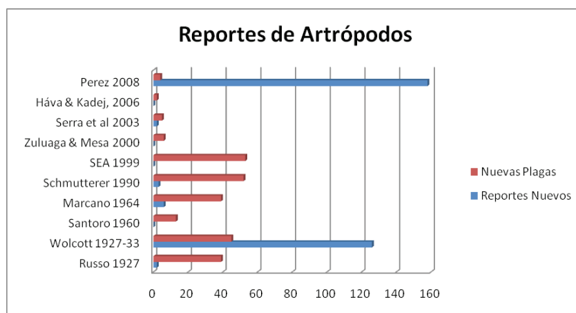
Fig. 1 Número de registros de artrópodos y plagas nuevas según Perez-Gelabert 2008
