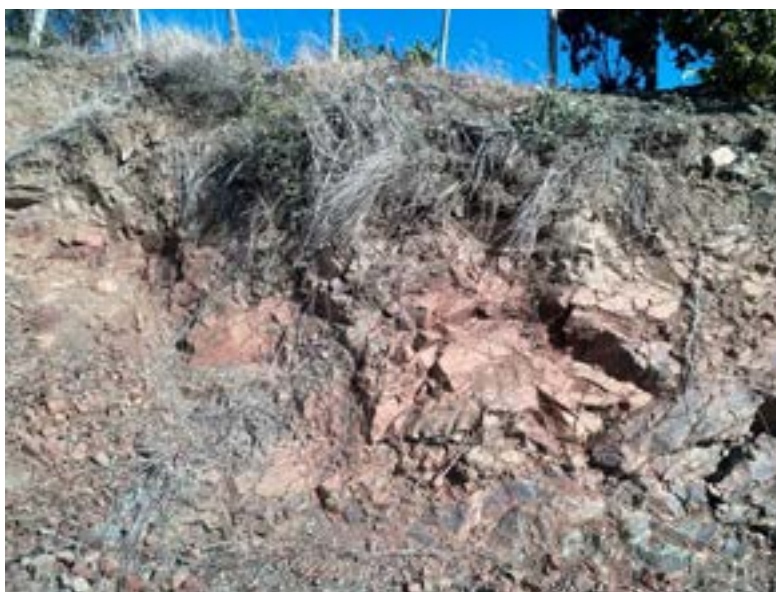
Figura 19. Perfil de suelo en sitios degradados con limitación en profundidad efectiva.
