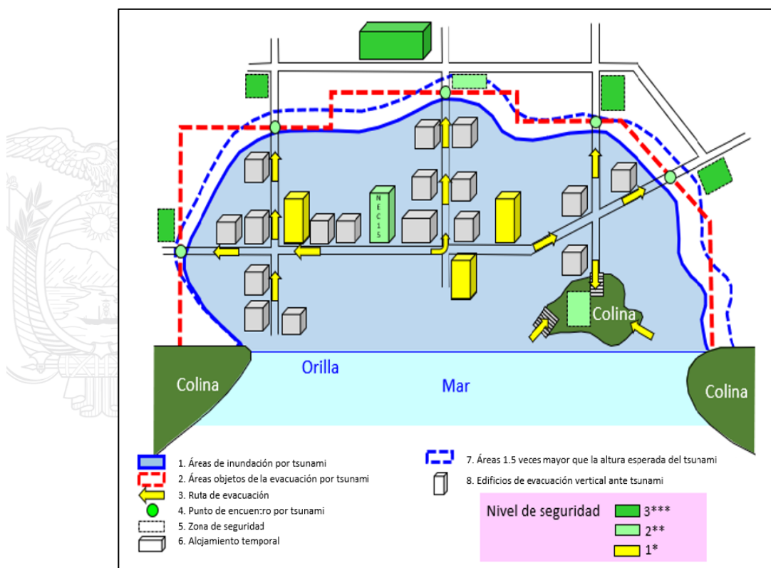
Ilustración 25. Nivel de seguridad de edificios de evacuación vertical ante tsunami
