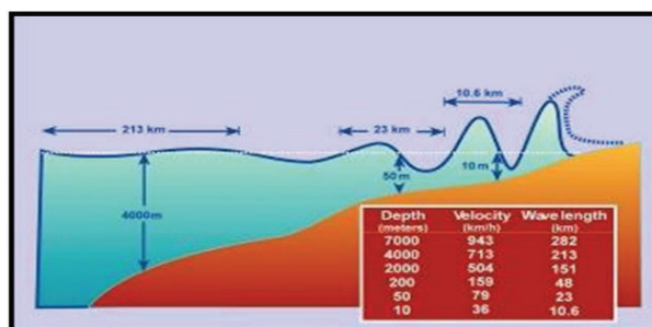
Ilustración 1. Velocidad y altura de la ola según la profundidad 2
