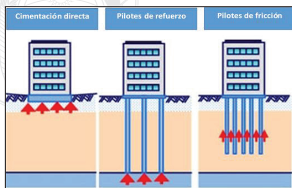
Ilustración 20. Tipo de cimentación de los edificios
