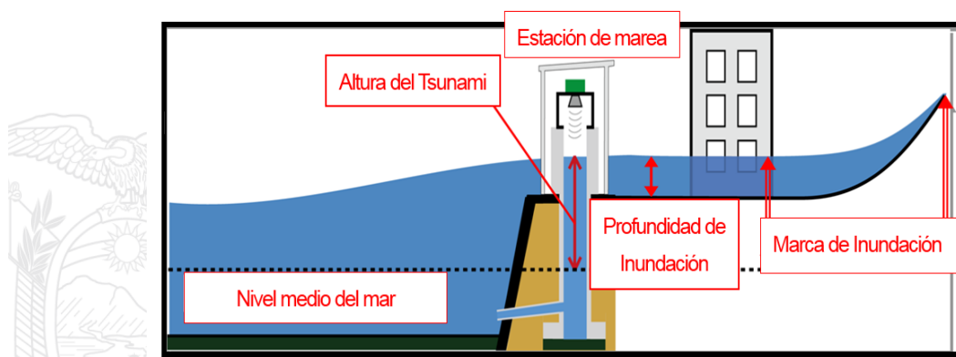
Ilustración 2. Descripción gráfica de la terminología de tsunami
