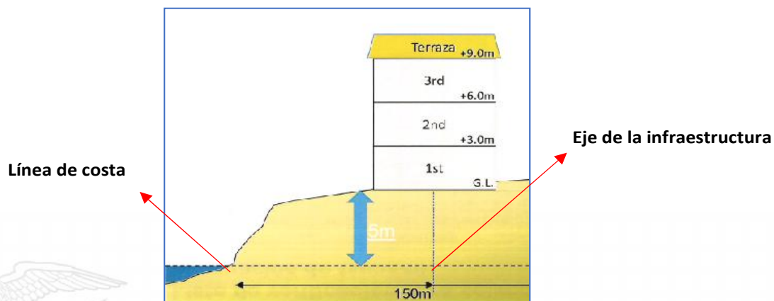
Ilustración 2: Distancia línea de costa a eje infraestructura
