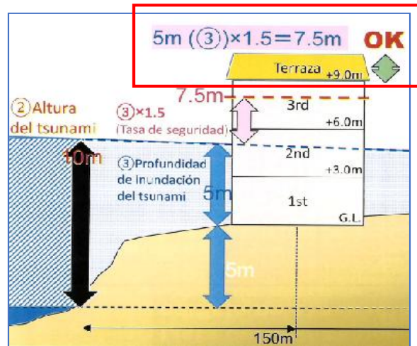
Ilustración 9: Esquema de altura de 1,5 veces superior a la profundidad de inundación del tsunami
