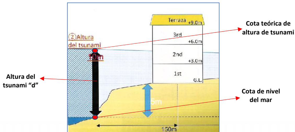
Ilustración 6: Esquema de altura del tsunami
