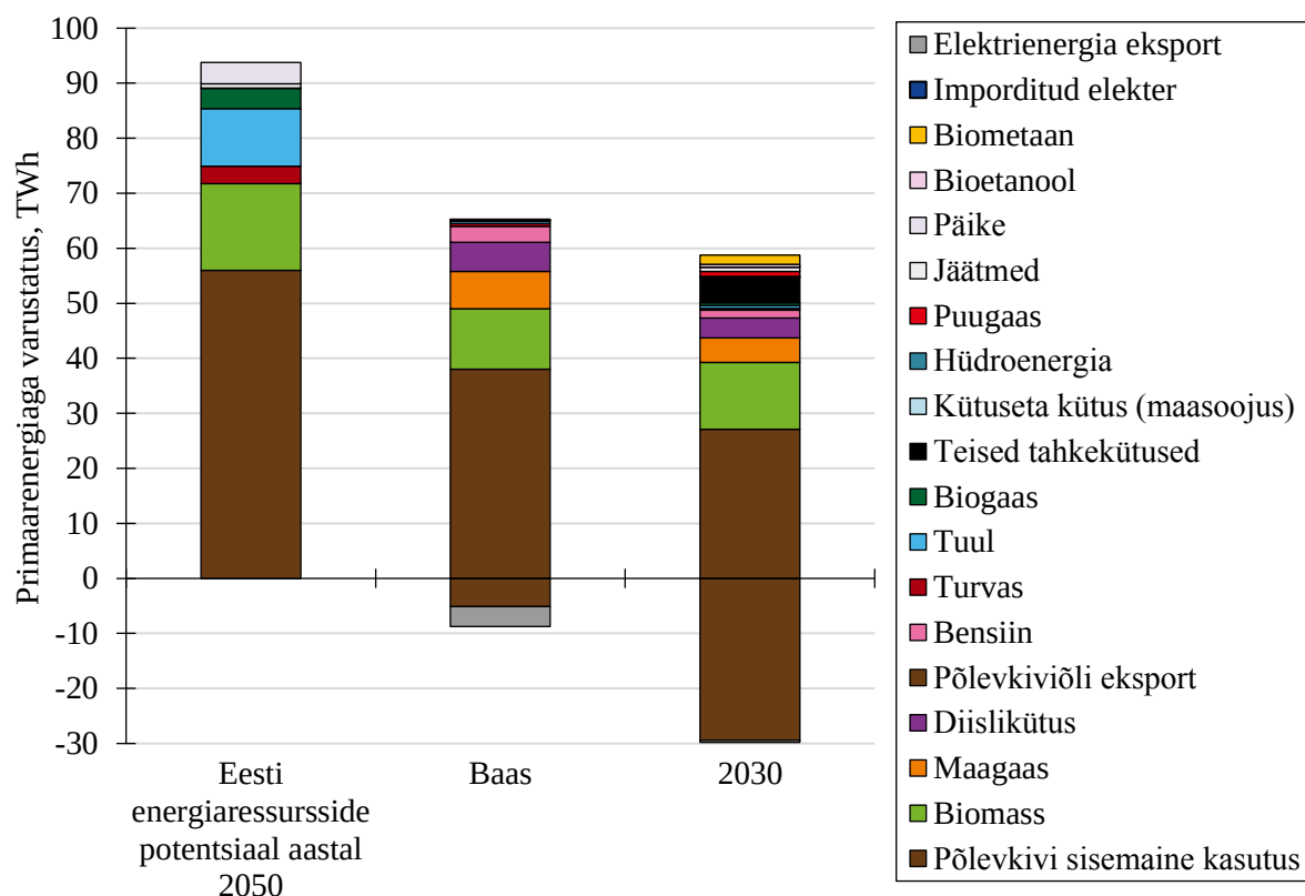
Joonis 3.26. Eesti primaarenergia allikate potentsiaal ja kasutamise prognoos energia muundamisel (sh import ja eksport) 60, 61
