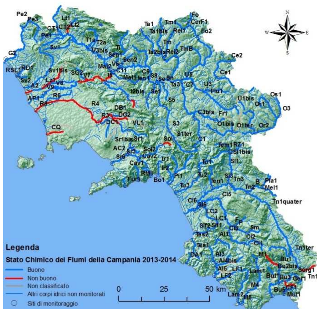
Figura 3.1.4.2_Rappresentazione dello Stato Chimico dei fiumi Campani 2013-2014
