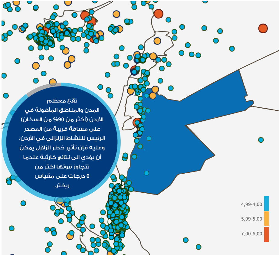
الشكل 3: توزع الزلازل على طول الصدع التحويلي الأردني خلال الفترة 1900 - 2005 (المصدر: مرصد الزلازل الأردني، 2007)
