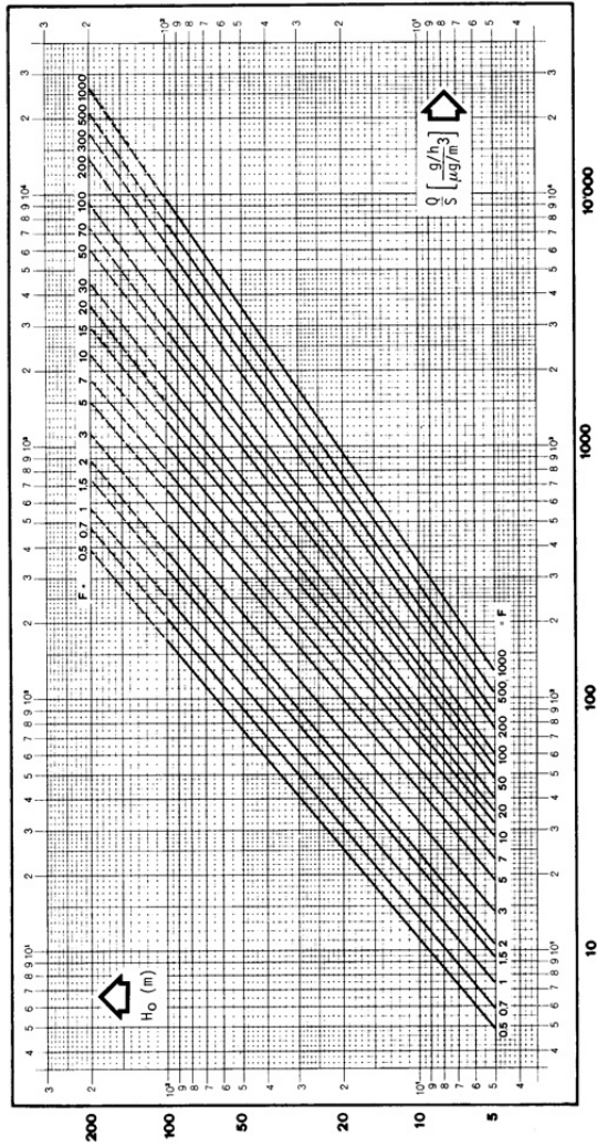
Bestimmung der Rechengröße H_0 für Hochkamine
