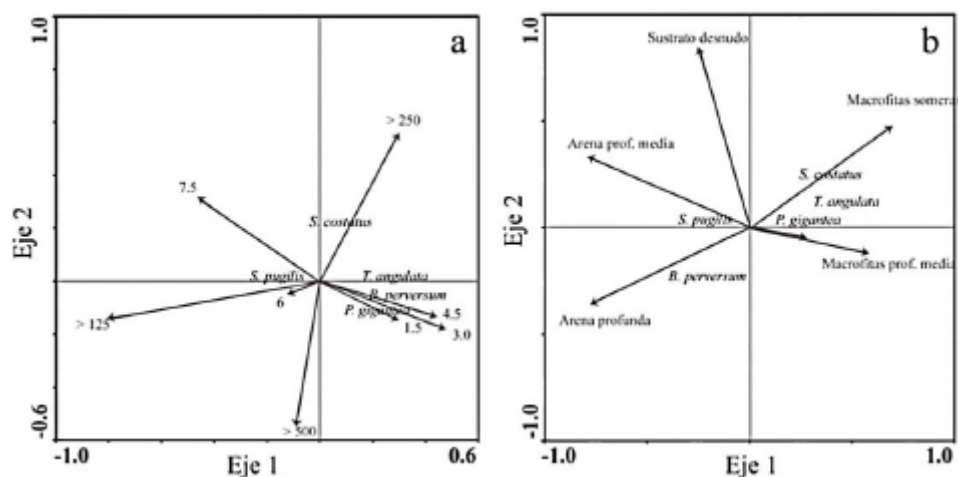
Figura 22. Análisis de correspondencia canónica (CCA), donde se muestra la asociación estadística entre las especies de gasterópodos con las variables en sedimento (a: > 125 = arena fina, >250 = arena media, >500 = arena gruesa. 1.5, 3, 4.5, 6 y 7.5 = porcentaje de materia orgánica) y entre las especies con los tipos de fondo (b), basados en los primeros ejes canónicos.
