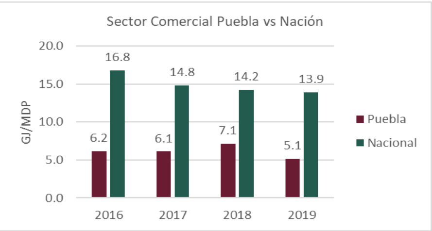
Figura 4.5 Comparación de la intensidad energética del sector comercial de Puebla vs nacional. (GJ/ MDP)
