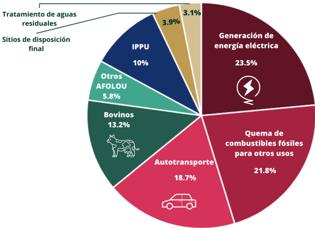
Figura 3.6 Principales categorías de emisiones de GEI en México, 2019
