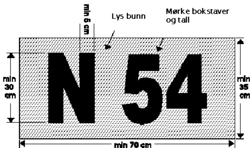
Figur 6. Merke for kilenot og lakseverp.
