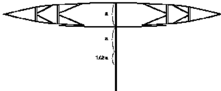
Figur 10. Stengingsmåte nr. 2 for dobbel kilenot.
