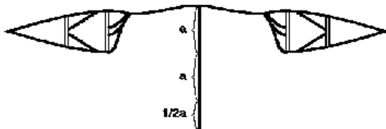
Figur 9. Stengingsmåte nr. 1 for dobbel kilenot.
