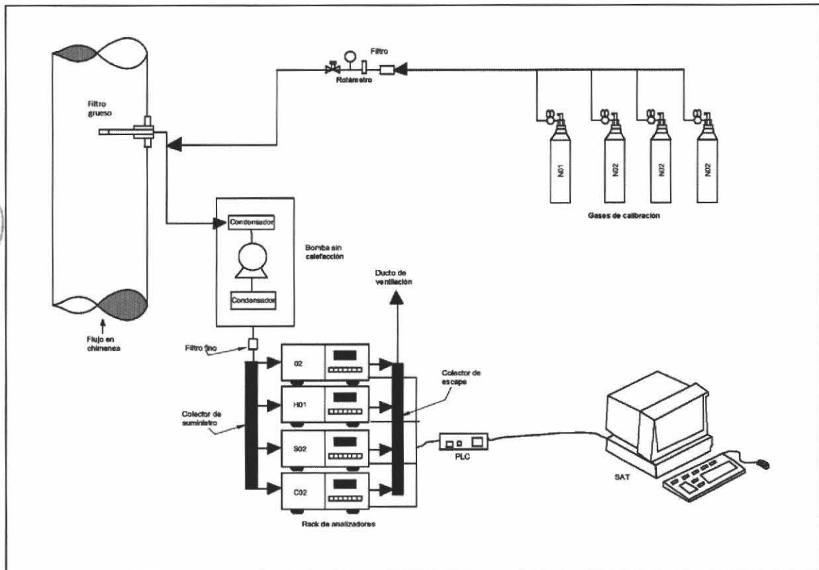
FIGURA N° 6 CEMS EXTRACTIVO DIRECTO: SISTEMAS FRÍO - SECO
