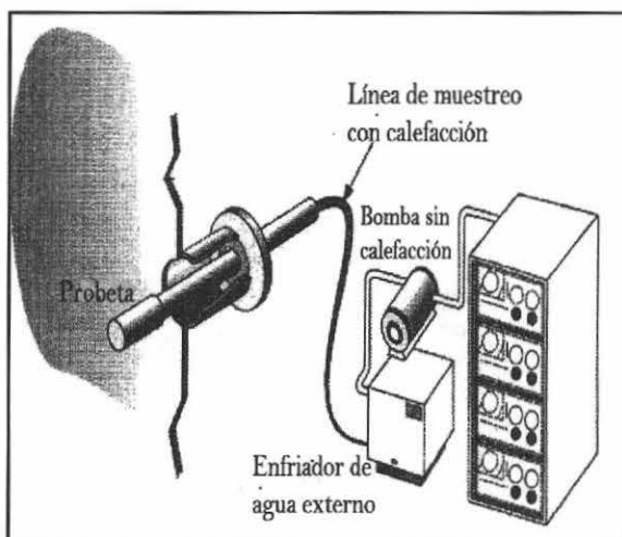
FIGURA N°5 ESQUEMA DE LOS TIPOS DE EXTRACCIÓN
