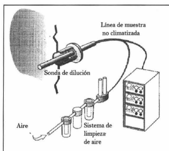
FIGURA N°5 ESQUEMA DE LOS TIPOS DE EXTRACCIÓN
