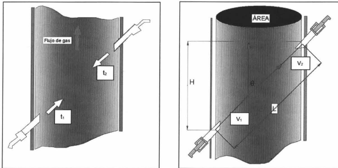
FIGURA N°9 GEOMETRÍA DE LA CHIMENEA
