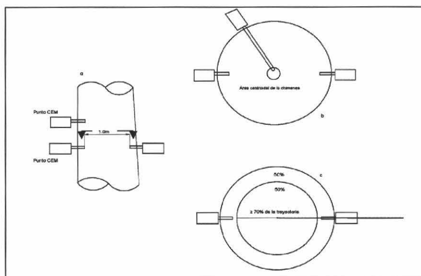
FIGURA N°2 UBICACIÓN DEL PUNTO DE MEDICIÓN
