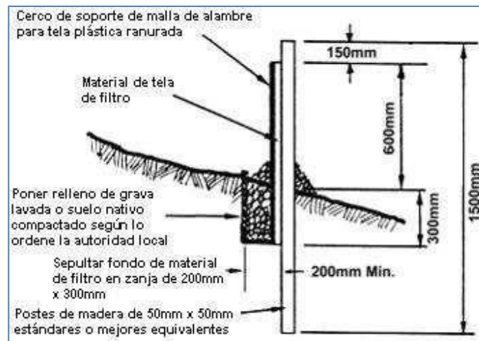
Figura N° 11. Detalle de cerco de tela de filtro
