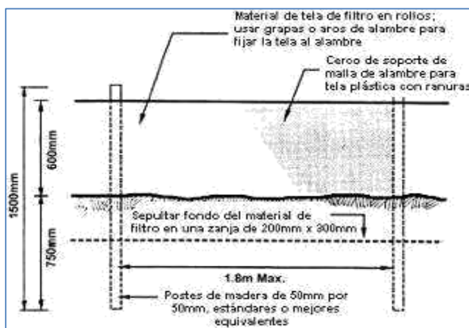
Figura N° 10. Detalle de cerco de tela de filtro
