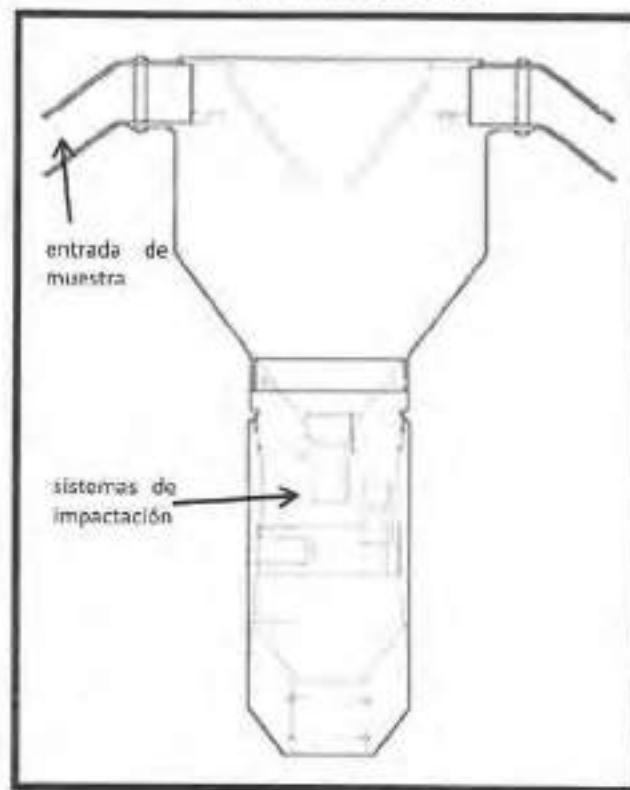
Figura 5. Esquema de un cabezal selectivo de bajo volumen para PM_{10}
