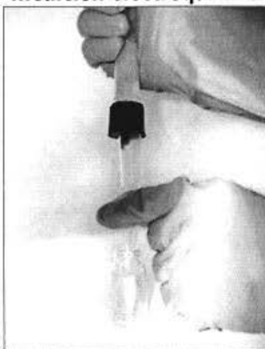
Figura N° 8: Extracción de solución acuosa con iones de cloro para su medición electroquímica
