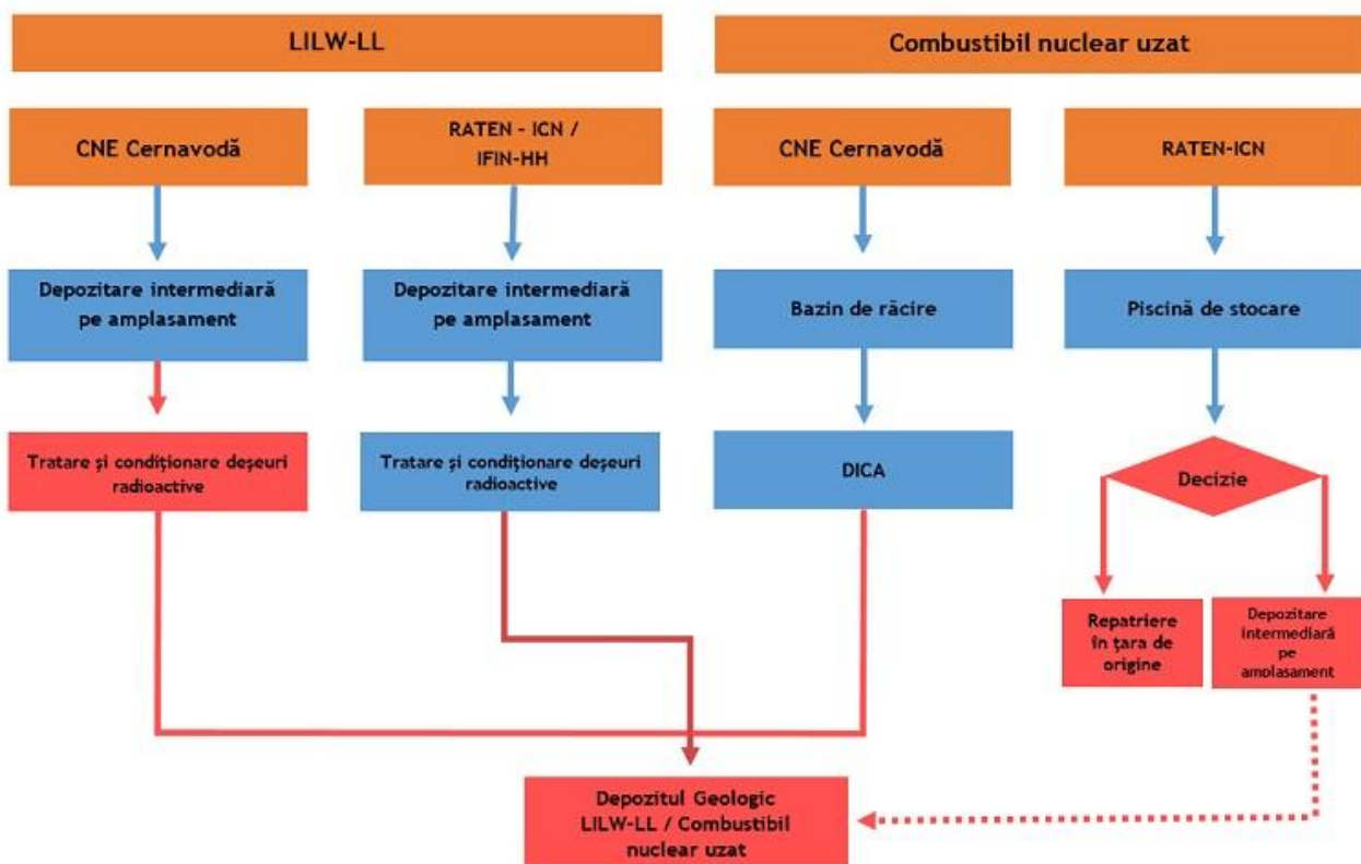
Figura 2 - Diagrama managementului combustibilului nuclear uzat și a deșeurilor
