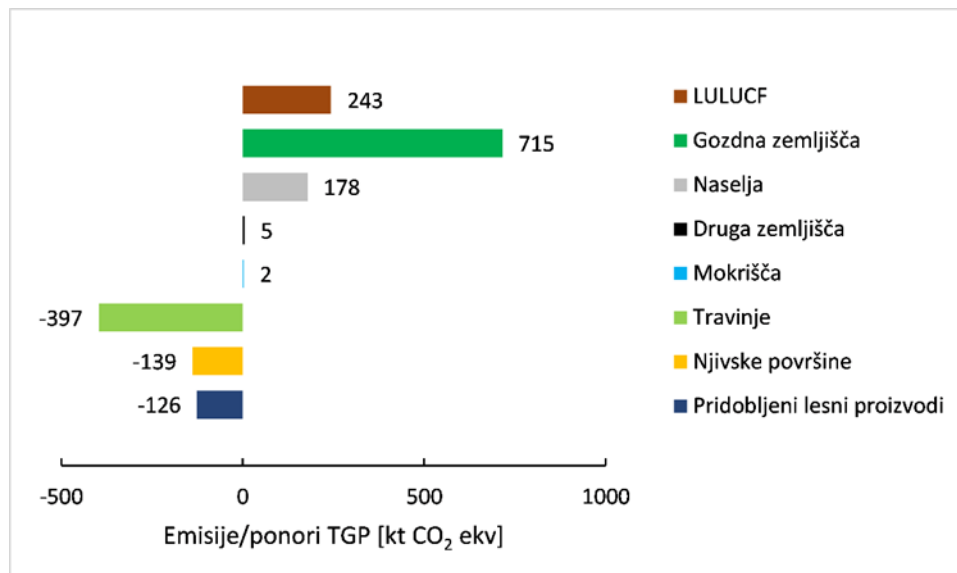
Slika 17: Bilanca emisij in ponorov TGP sektorja LULUCF v letu 2018 (vir: GIS)
