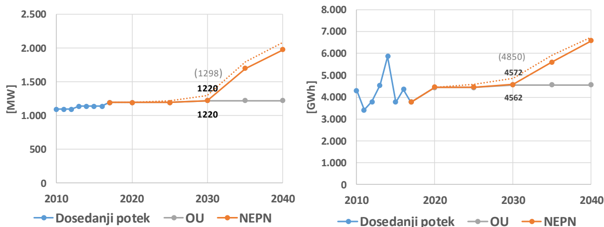
Slika 42: Razvoj velikih HE in čHE – instalirane kapacitete in proizvodnja elektrike na generatorju 80
