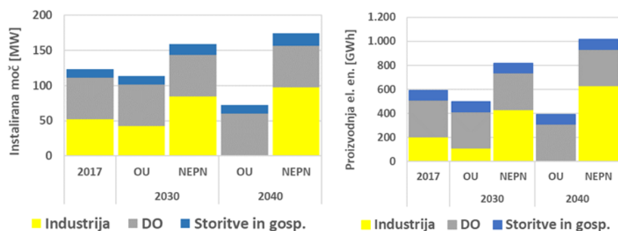
Slika 46: Projekcija instalirane moči in proizvodnja električne energije v sistemih SPT za scenarij z obstoječimi ukrepi in za scenarij NEPN
