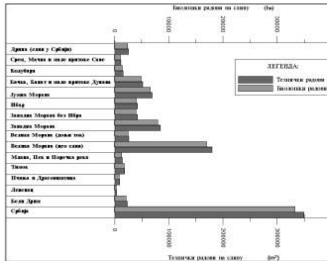
Слика 43. Обим противерозионих радова за одржавање постојећег стања ерозије у Републици Србији
