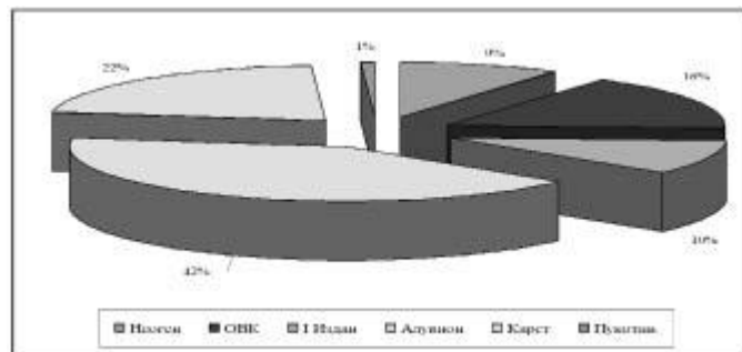
Слика 19. Заступљеност типова издани у снабдевању водом општинских центара (Извор: РЗС и ИЈЧ)
