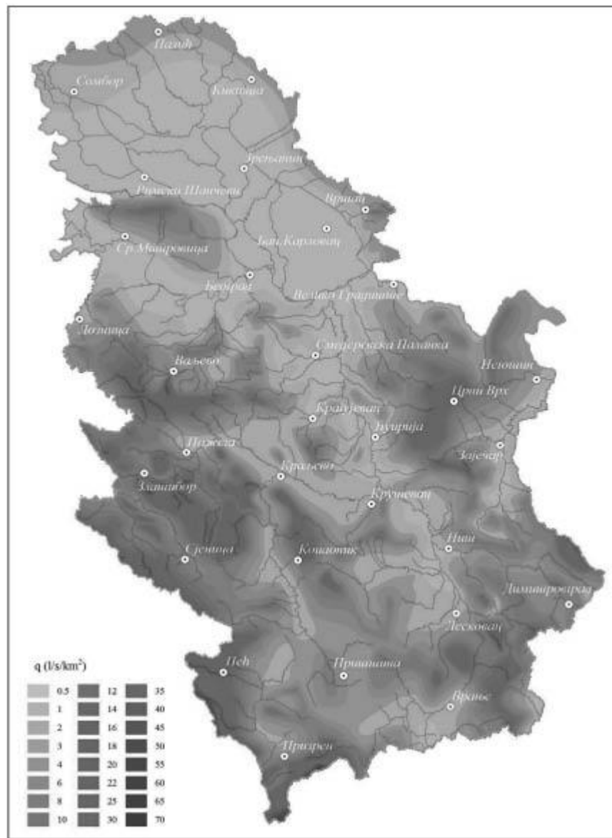
Слика 3. Модули отицаја (Извор: подаци РХМЗ-а)
