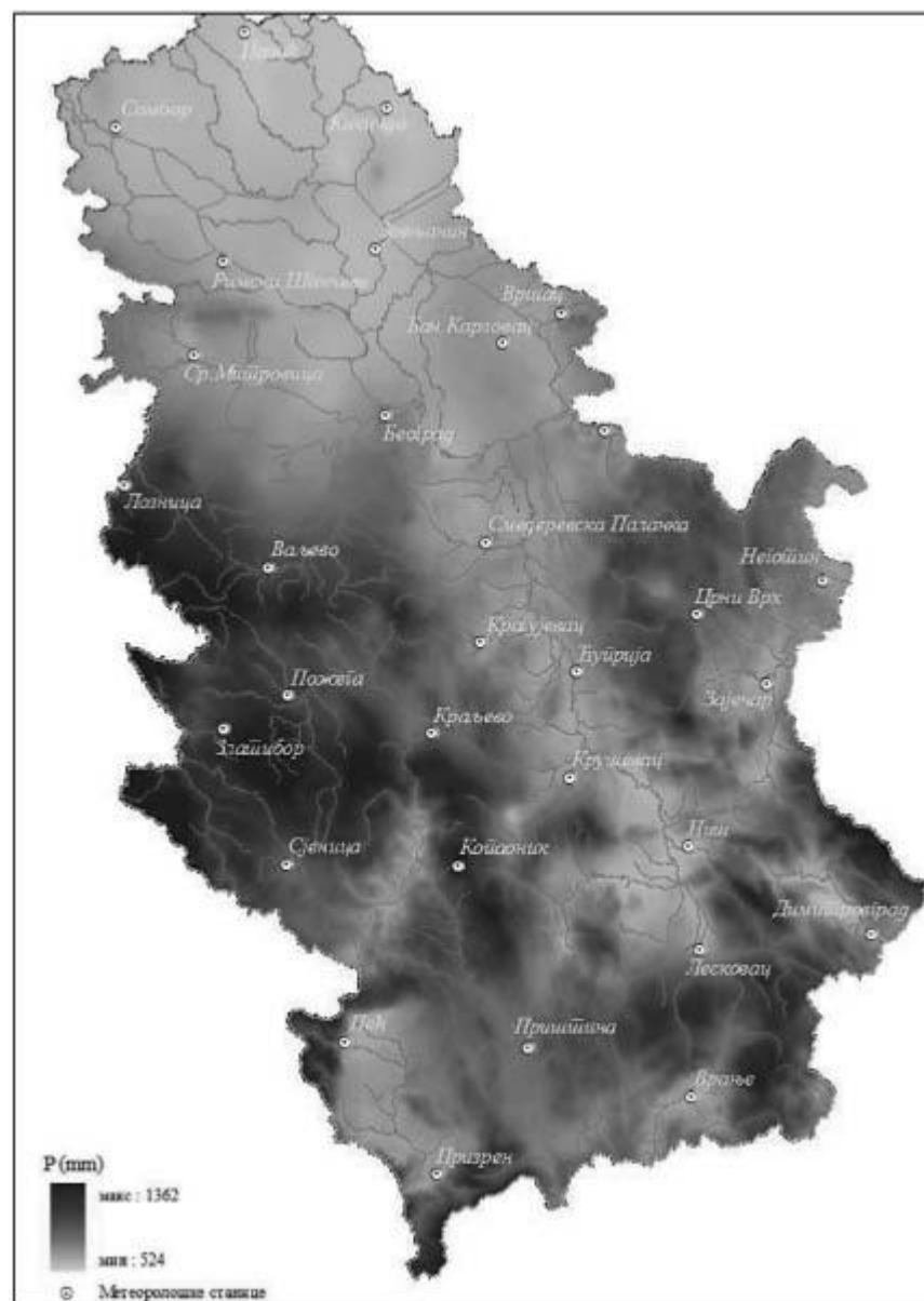
Слика 2. Просечне вишегодишње суме падавина (Извор: подаци РХМЗ-а)
