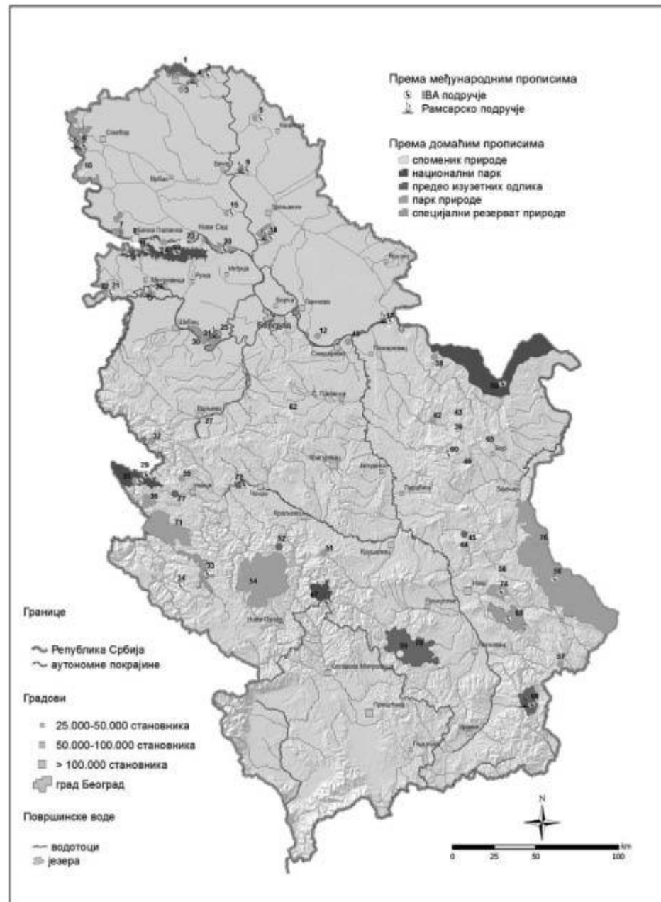
Слика 12. Заштићена подручја (Извор: документациона база ИЈЧ)
