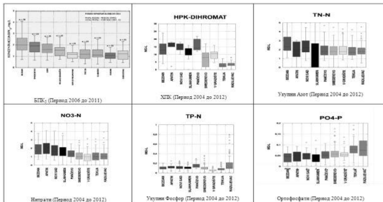
Слика 28. Опажени трендови квалитета воде дуж тока Дунава у Републици Србији Извор: ИЈЧ
