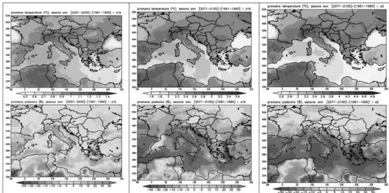
Слика 47. Годишња промена температуре и падавина у ближој (А1Б) и даљој будућности (А1Б и А2 сценарији) у односу на период 1961–1990. године
