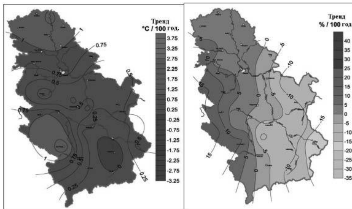
Слика 46. Годишњи температурни (слика лево) и падавински (слика десно) трендови у Републици Србији
