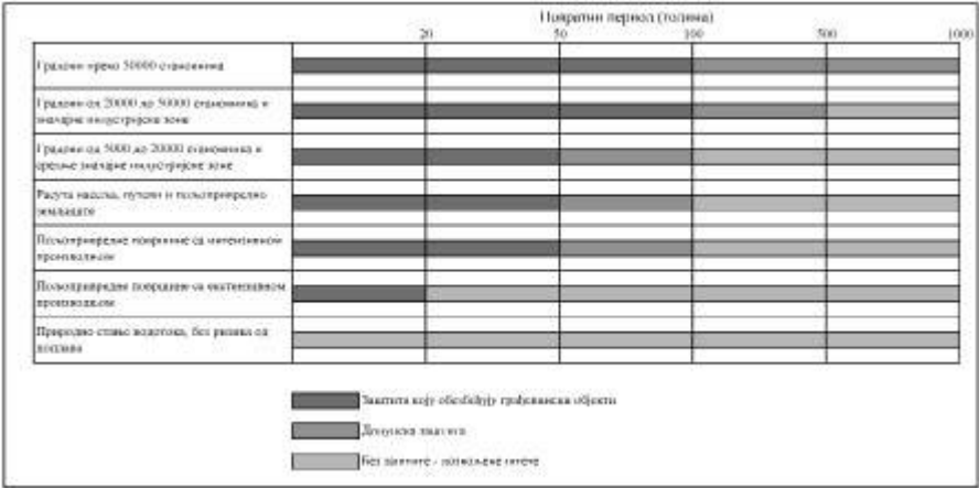
Слика 42. Препоручени степен заштите од поплава
