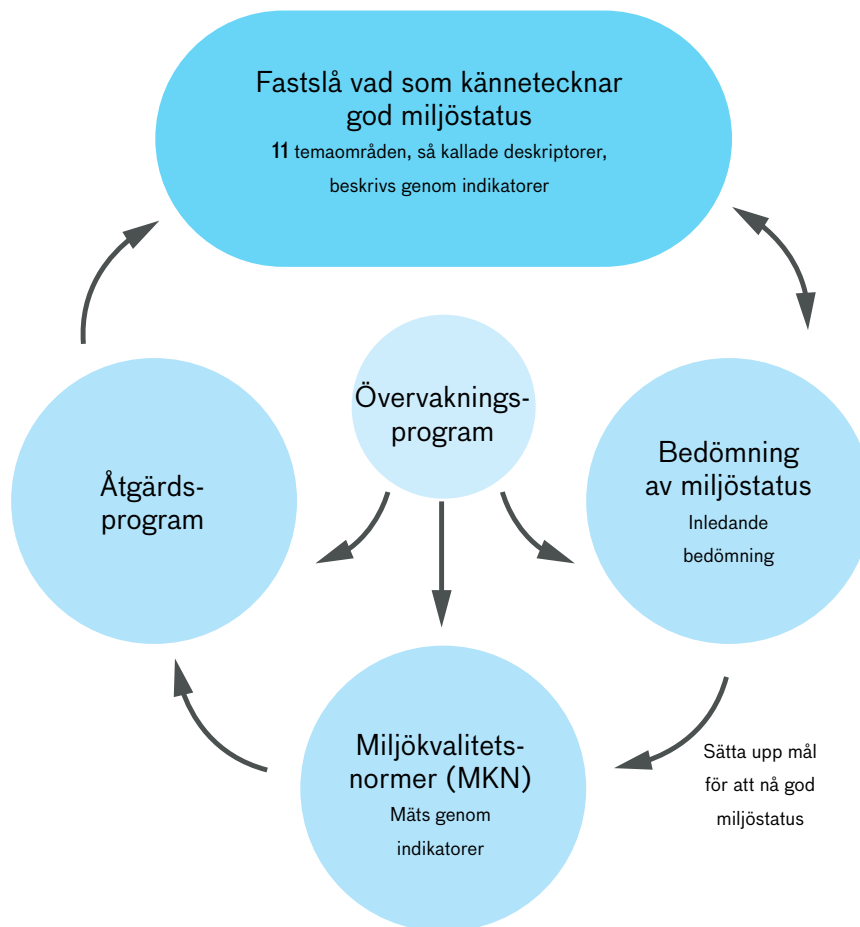
Figur 15. Översiktlig illustration av havsmiljöförordningens process och begrepp.
