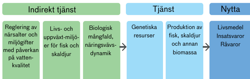
Figur 29. Viktiga ekosystemtjänster för yrkesfisket.
