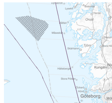
Figur 42. Gråmarkerat område markerar dumpningsområdet för vrak innehållande okända mängder kemiska stridsmedel. Kemiska stridsmedel har detekterats i biota och sediment på flertalet platser inom området.
