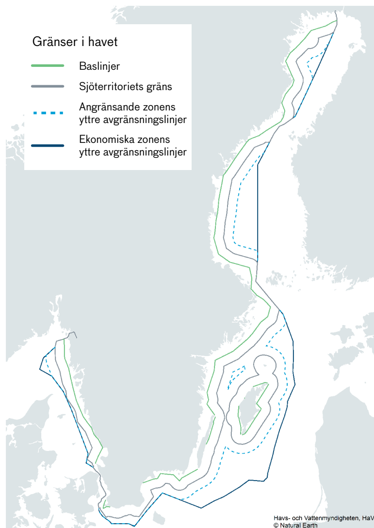
Figur 3. Gränser i havet
