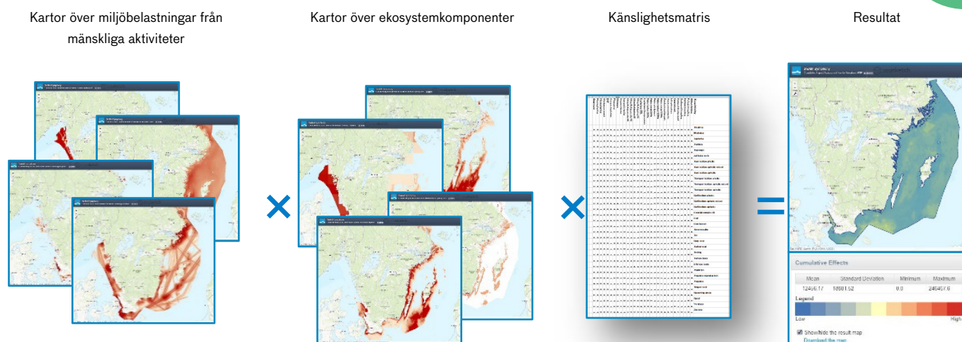
Figur 36. Metod för Symphony, kumulativ miljöpåverkan. Symphony beräknar summan av alla verksamheters påverkan på alla naturvärden med olika känslighet. Beräkningen görs på varje plats i havet, uppdelat i ett rutnät med rutor om 250 x 250 meter.
