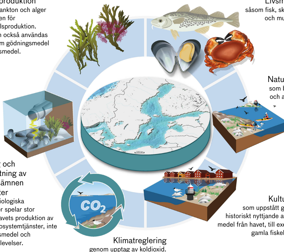
Figur 26. Havets ekosystem bidrar med flera samhällsviktiga funktioner som till exempel produktion av livsmedel. De mer synliga ekosystemtjänsterna påverkar och är beroende av andra indirekta som inte är så synliga. Till exempel är fiskar beroende av livskraftiga livsmiljöer och lekområden för att överleva och ge bärkraftiga fiskbestånd. Ett annat exempel är ekosystem som bryter ner näringsämnen och gifter.
