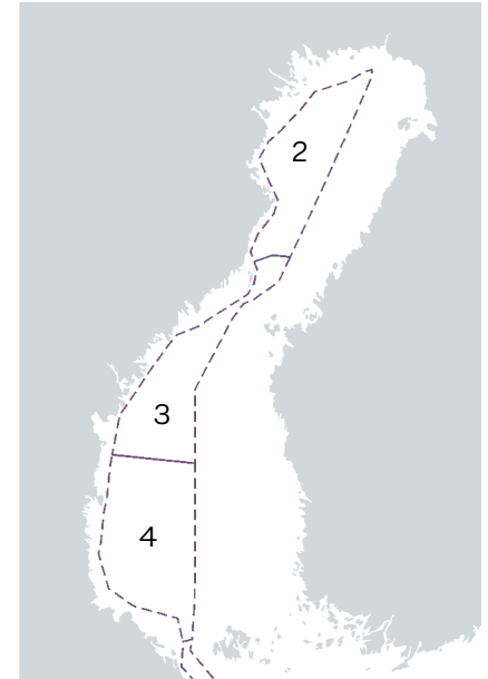
Figur 16. De tre havsområdena inom Bottniska viken. Numrering enligt kartnummer.
