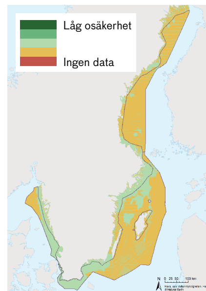
Figur 35. Symphony osäkerhetskarta. Medelvärde av osäkerhetsgrad.
