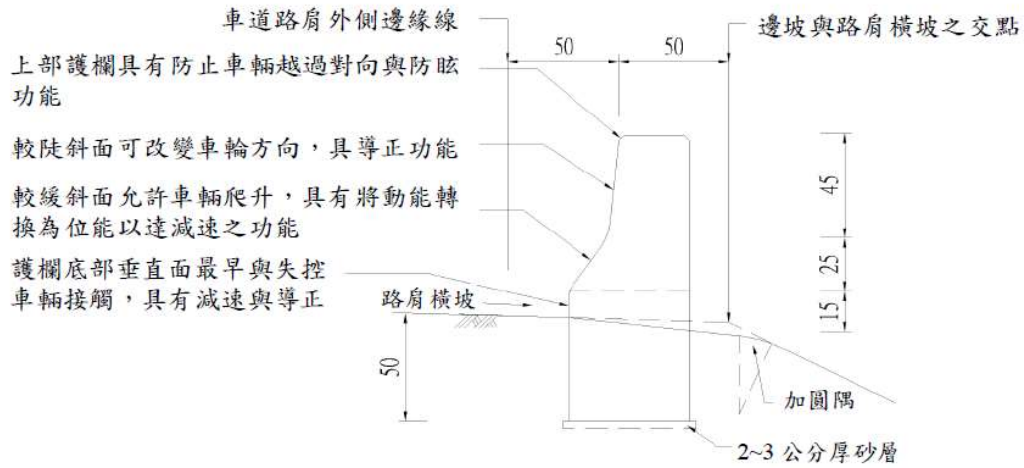
剖面圖
