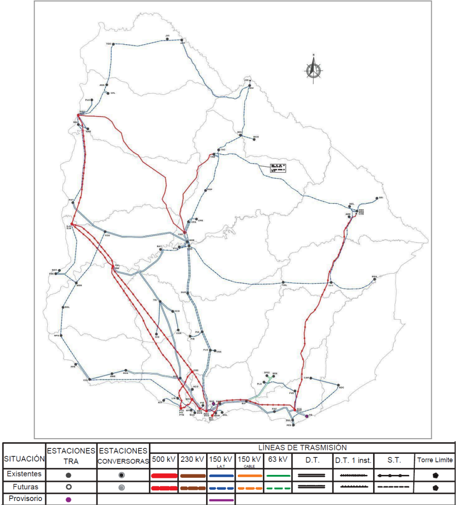
Figura 5 Mapa de líneas de transmisión gestionadas por UTE y Salto Grande mayores a 60kV – Fuente: Memoria anual UTE, 2022.
