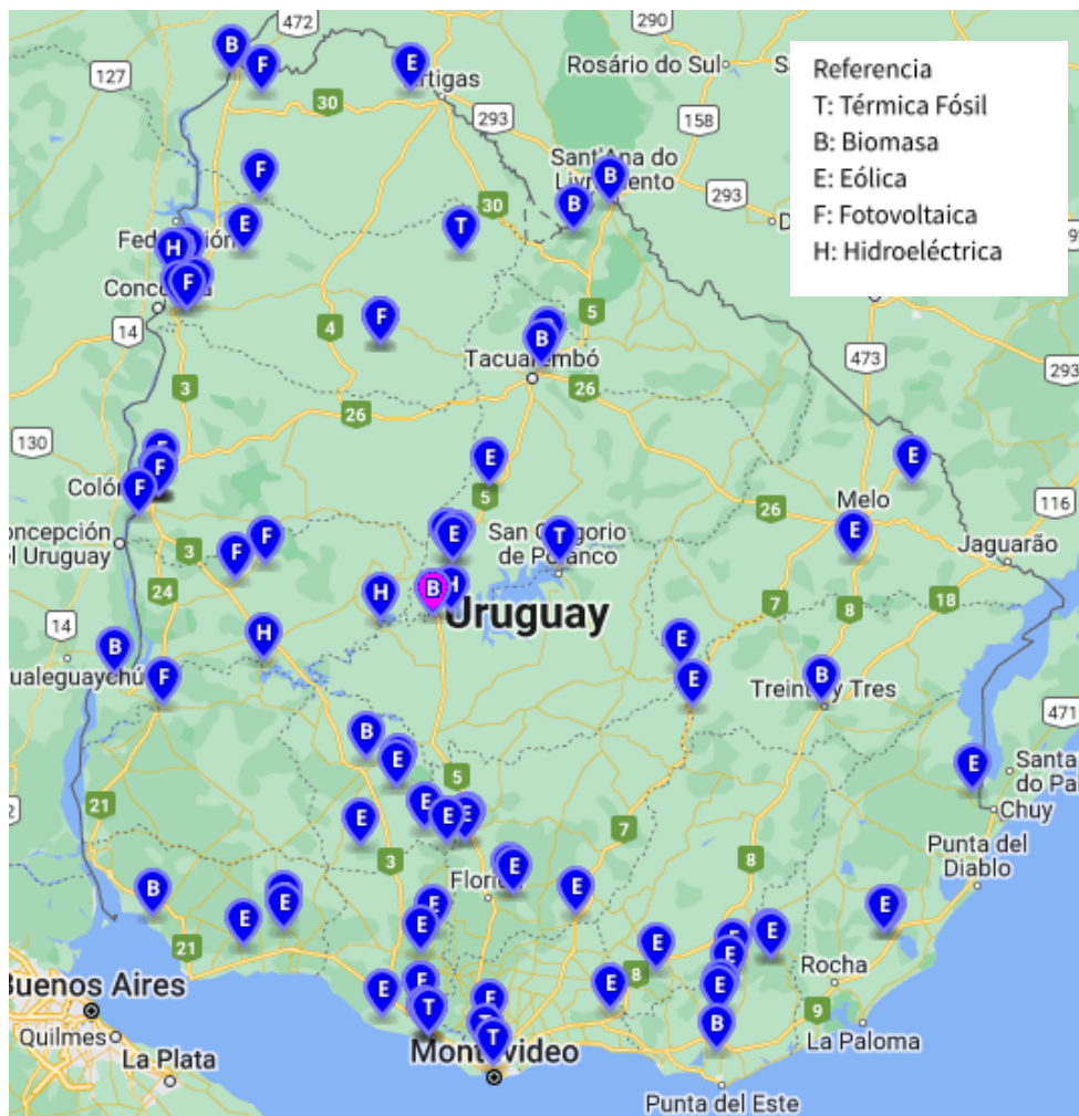
Figura 4 Generadores de energía eléctrica. 22
