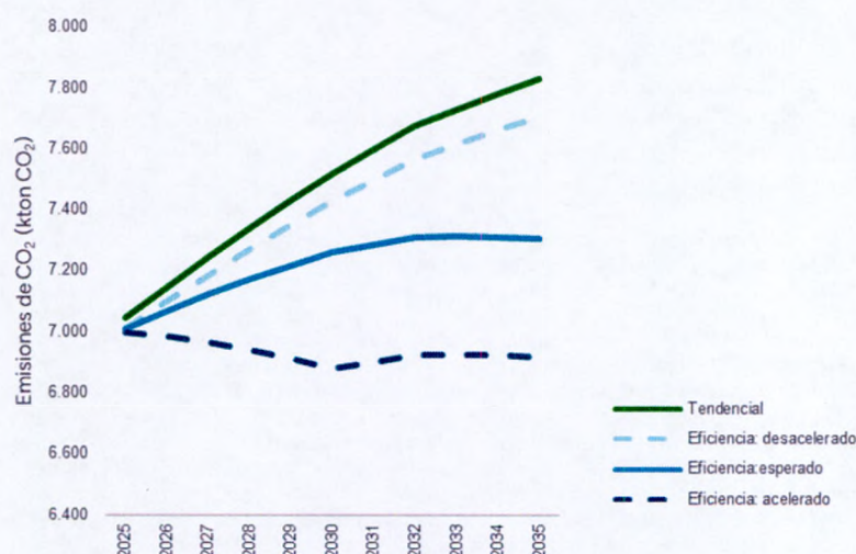
Figura 3. Escenarios de emisiones de \text{CO}_2 .
