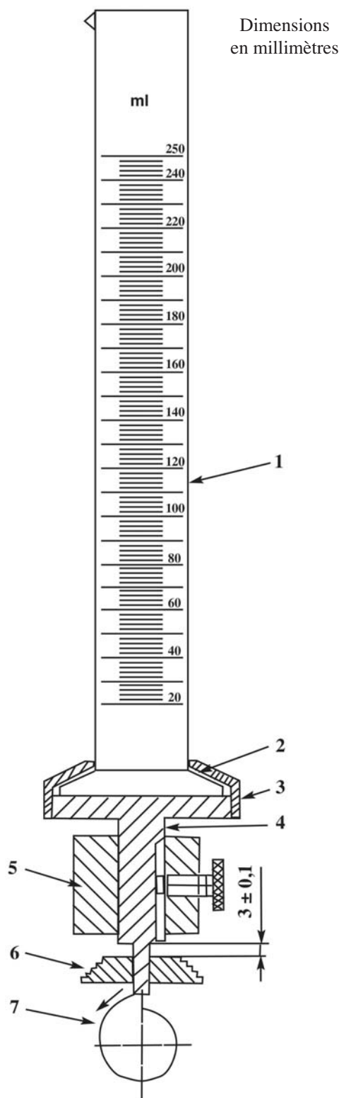
Figure : Appareil de mesure de la masse volumique
