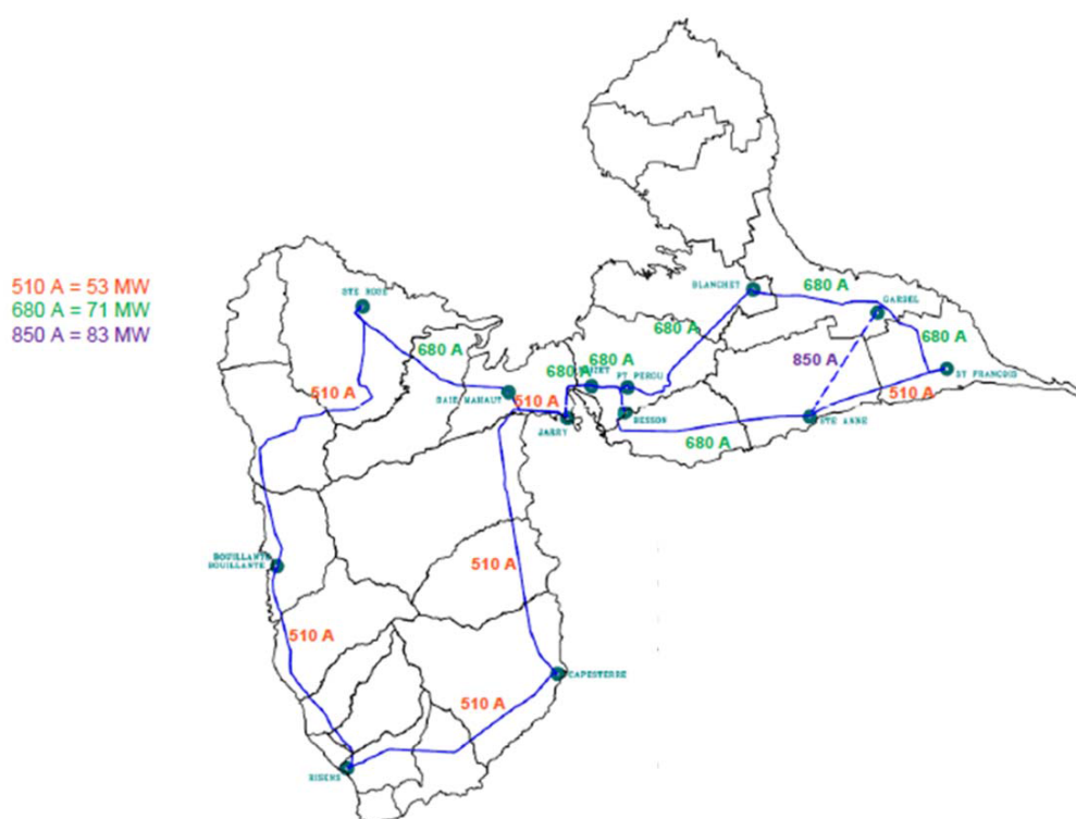
Figure 78 : Schéma du système électrique de transport guadeloupéen (EDE SEI)
