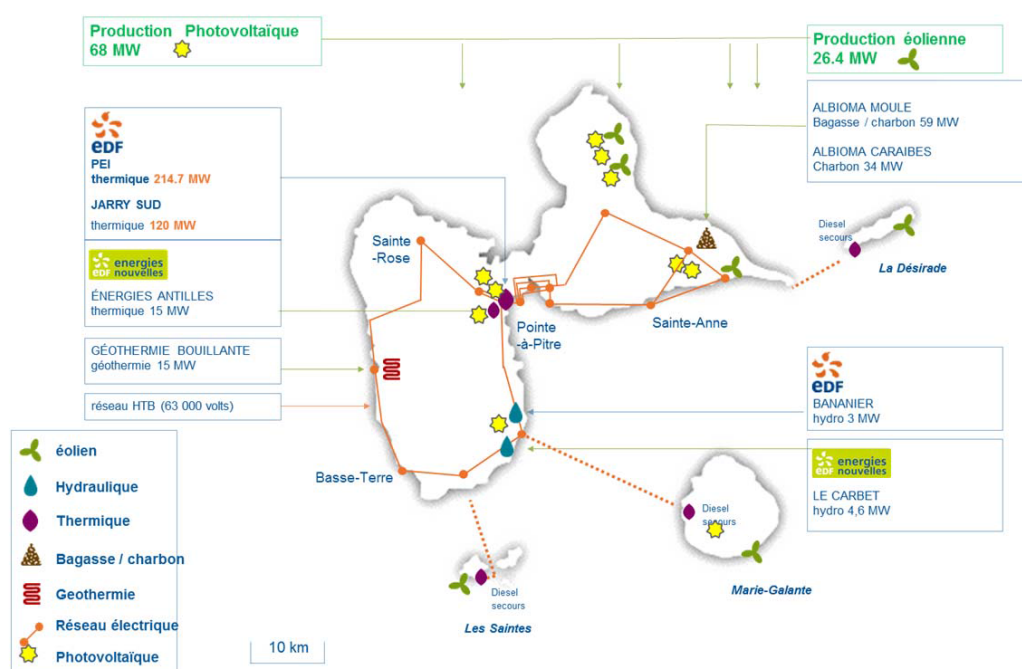
Figure 6 : Principales composantes du système électrique de la Guadeloupe en 2016 (EDF Archipel Guadeloupe)
