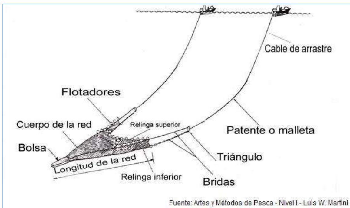
Figura 5 b. Pesca al arrastre de fondo a la pareja
