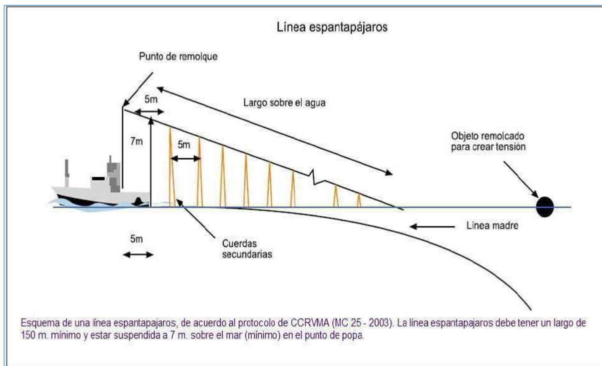
Figura 17 a: Esquema de la línea espantapájaros
