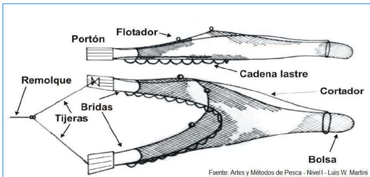
Figura 8 b: Aparejo de un Buque tangonero
