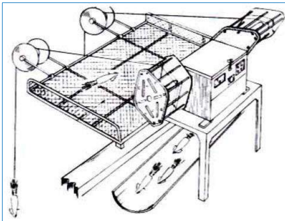
Figura 10 c: Esquema de las máquinas calamareras automática
