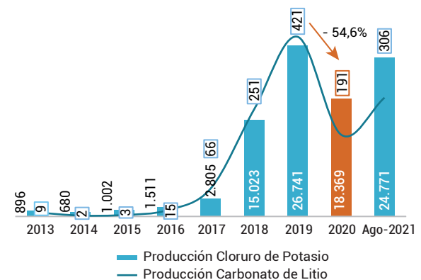
Bolivia: Producción de Carbonato de Litio y Cloruro de Potasio, 2013 - Agosto 2021 (En toneladas métricas)
