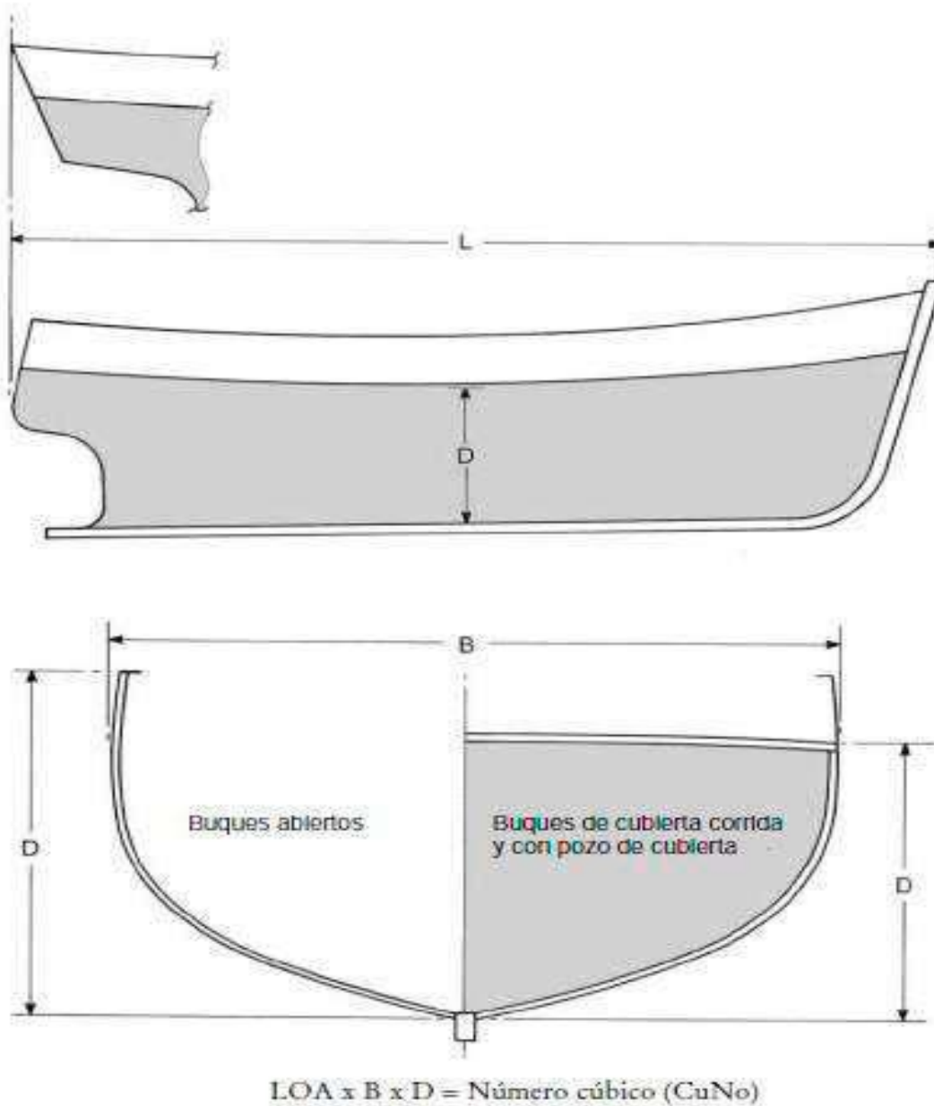
Figura 6 Número cúbico
