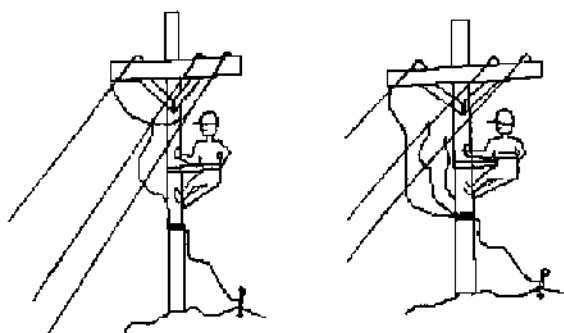
Figura 15. Montajes típicos de puestas a tierra temporales.
