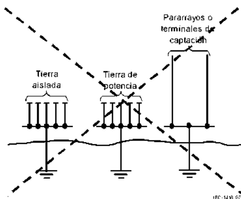
Figura 12. Puestas a tierra separadas o independientes (prohibido).
