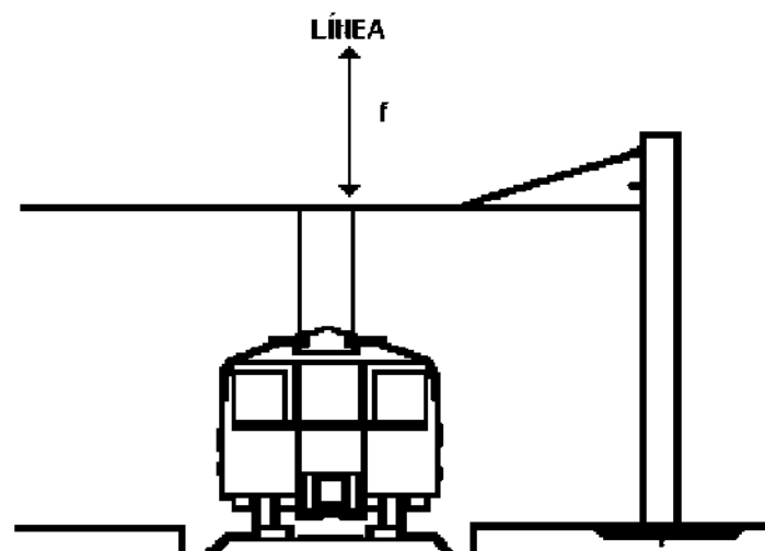
Figura 8. Distancia "f" en cruces con ferrocarriles electrificados.
