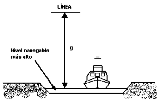
Figura 9. Distancia "g" en cruces con ríos, cauces de agua, canales navegables
