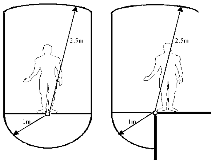
Figura 21. Distancias de seguridad contra contactos directos.
