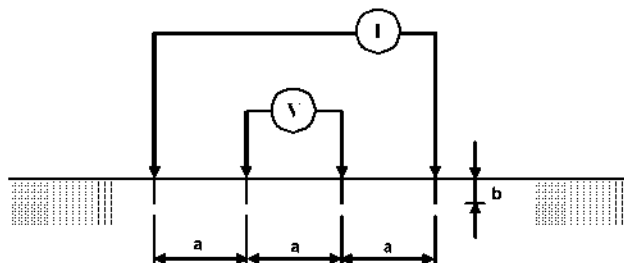
Figura 13. Esquema de medición de resistividad aparente.
