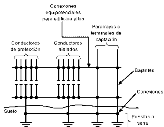
Figura 10. Sistemas con Puestas a tierra dedicadas e interconectadas.
