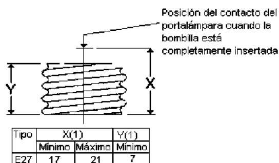
Figura 16. Posición de la camisa roscada del portalámpara. Las dimensiones están en mm.
