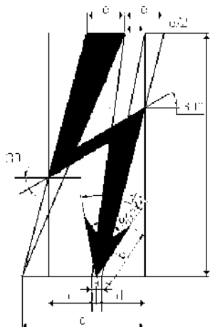
Figura 4. Símbolo de riesgo eléctrico No. 56 IEC 60417-1.
