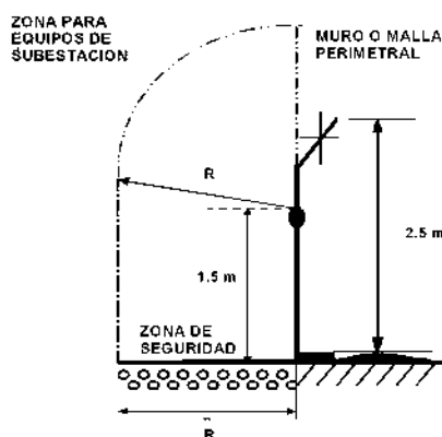
Figura 20. Zona de seguridad.
