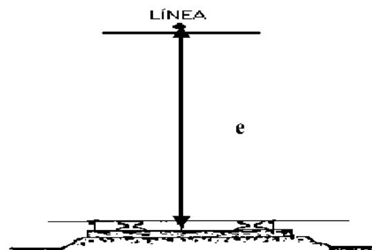
Figura 7. Distancia "e" en cruces con ferrocarriles sin electrificar
