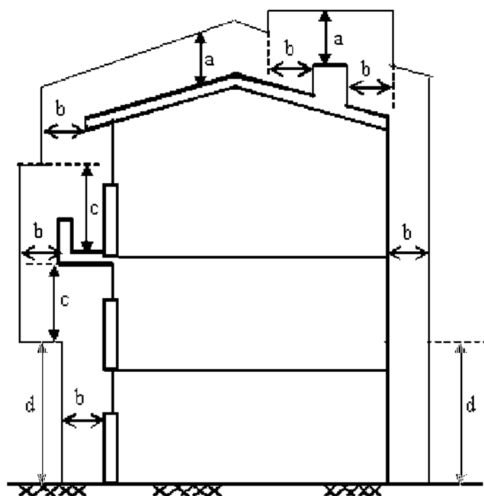
Figura 5. Distancias de seguridad en zonas con construcciones
