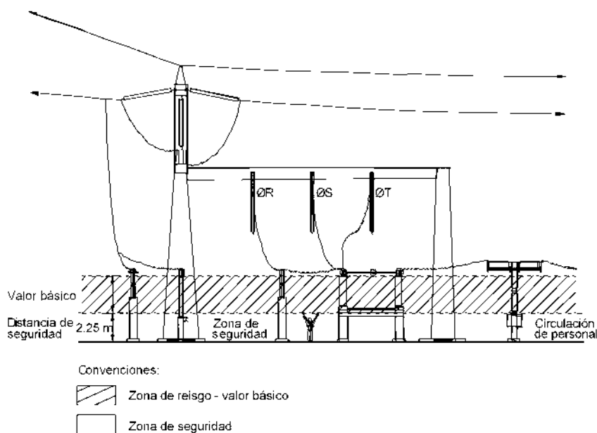
Figura 20. Zona de seguridad circulación de personal
