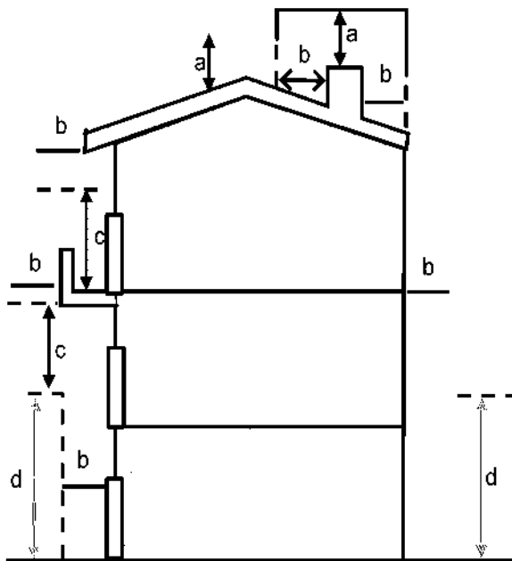
Figura 5. Distancias de seguridad en zonas con construcciones
