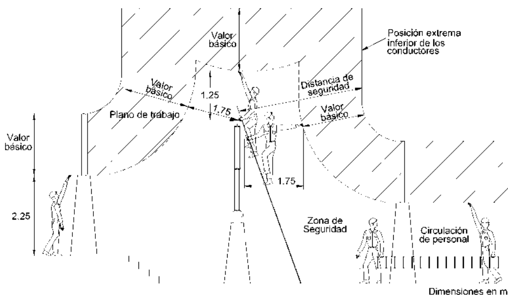
Figura 20. Zona de seguridad circulación de personal
