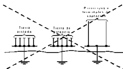
Figura 12. Puestas a tierra separadas o independientes
