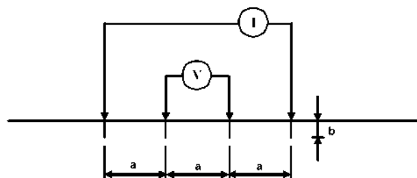
Figura 13. Esquema de medición de resistividad aparente.
