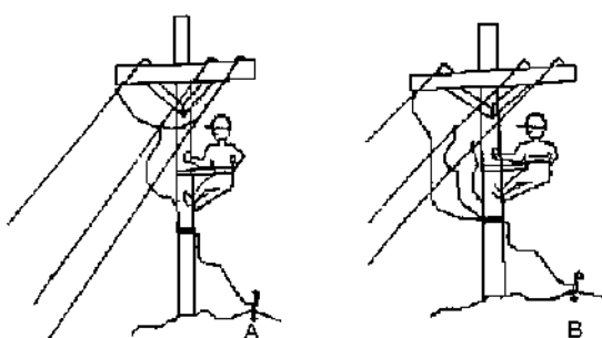
Figura 15. Montajes típicos de puestas a tierra temporales.
