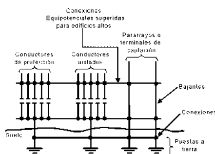
Figura 10. Sistemas con puestas a tierra dedicadas e interconectadas.
