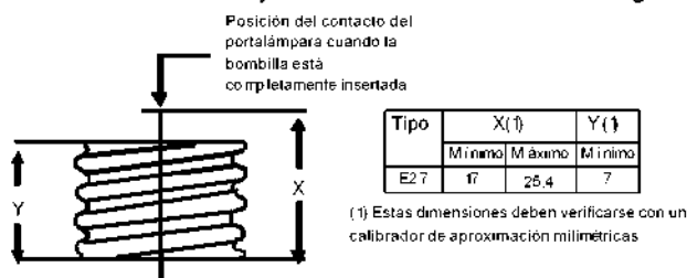
Figura 16. Posición de la camisa roscada del portalámpara. Dimensiones en milímetros.
