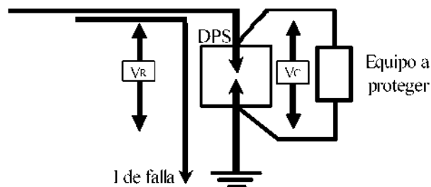
Figura 18. Montaje de los DPS
