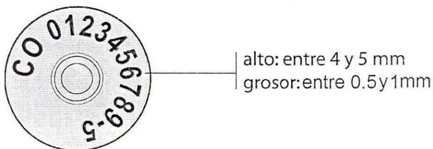
Gráfica 9. Imagen del anverso de la pieza hembra de la orejera tipo botón con radiofrecuencia.
