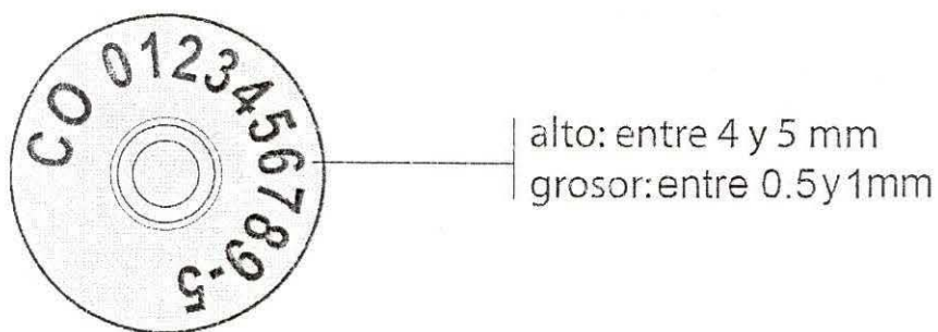
Gráfica 25. Imagen del anverso de la pieza hembra de la orejera tipo botón sin radiofrecuencia.
