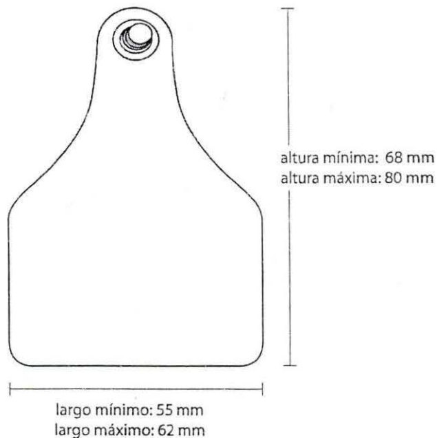
Gráfica 15. Imagen del anverso de la pieza hembra de la orejera tipo paleta sin radiofrecuencia.
