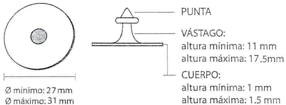
Gráfica 24. Dimensiones de la pieza macho de la orejera tipo botón sin radiofrecuencia.
