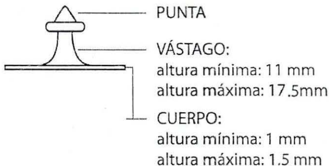
Gráfica 8. Dimensiones de la pieza macho de la orejera tipo botón con radiofrecuencia.
