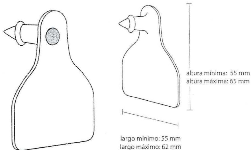
Gráfica 19. Imagen de la pieza macho tipo paleta de la orejera tipo paleta sin radiofrecuencia.
