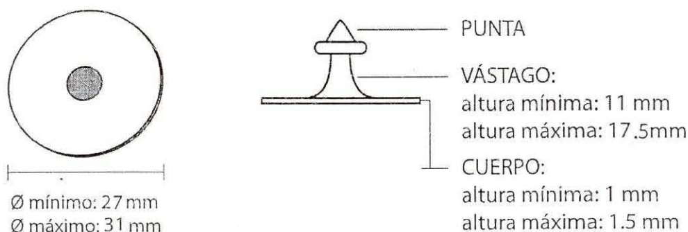
Gráfica 16. Imagen de la pieza macho circular de la orejera tipo paleta sin radiofrecuencia.
