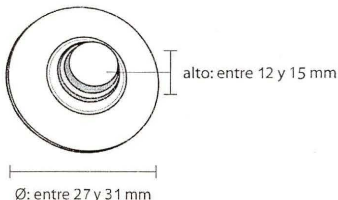
Gráfica 23. Dimensiones de la pieza hembra de la orejera tipo botón sin radiofrecuencia.
