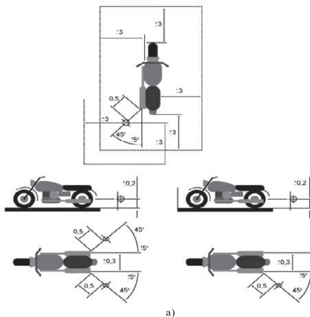
FIGURA 2. POSICIONES DEL SONÓMETRO SEGÚN EL TIPO DE VEHÍCULO (Dimensiones en metros, a menos que se indique lo contrario)
