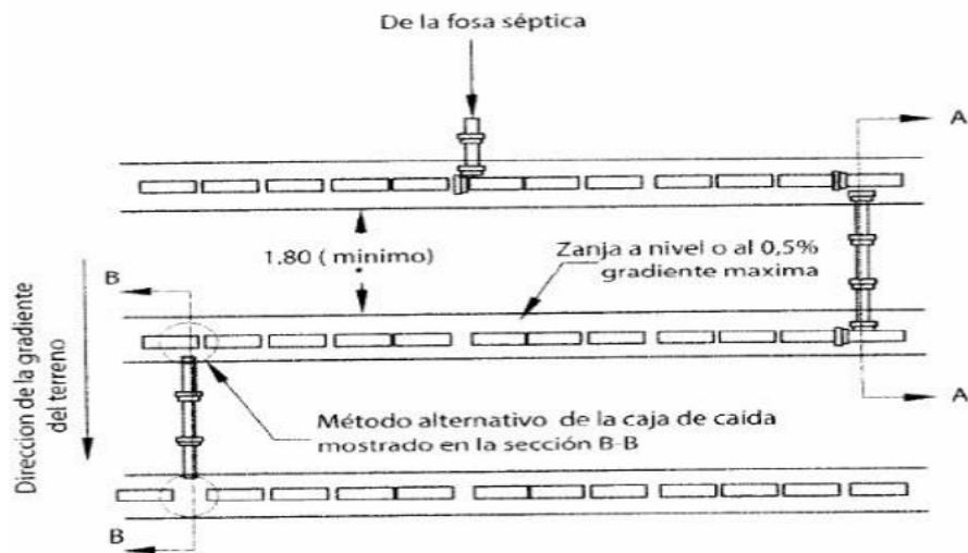
Figura D. Detalle constructivo de zanja de infiltración en terrenos inclina
