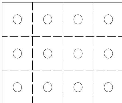
Figura 3. Ejemplo de puntos de medición de emisiones al aire en conducto de sección rectangular (12 áreas iguales con punto de medición en centroide de cada área).
