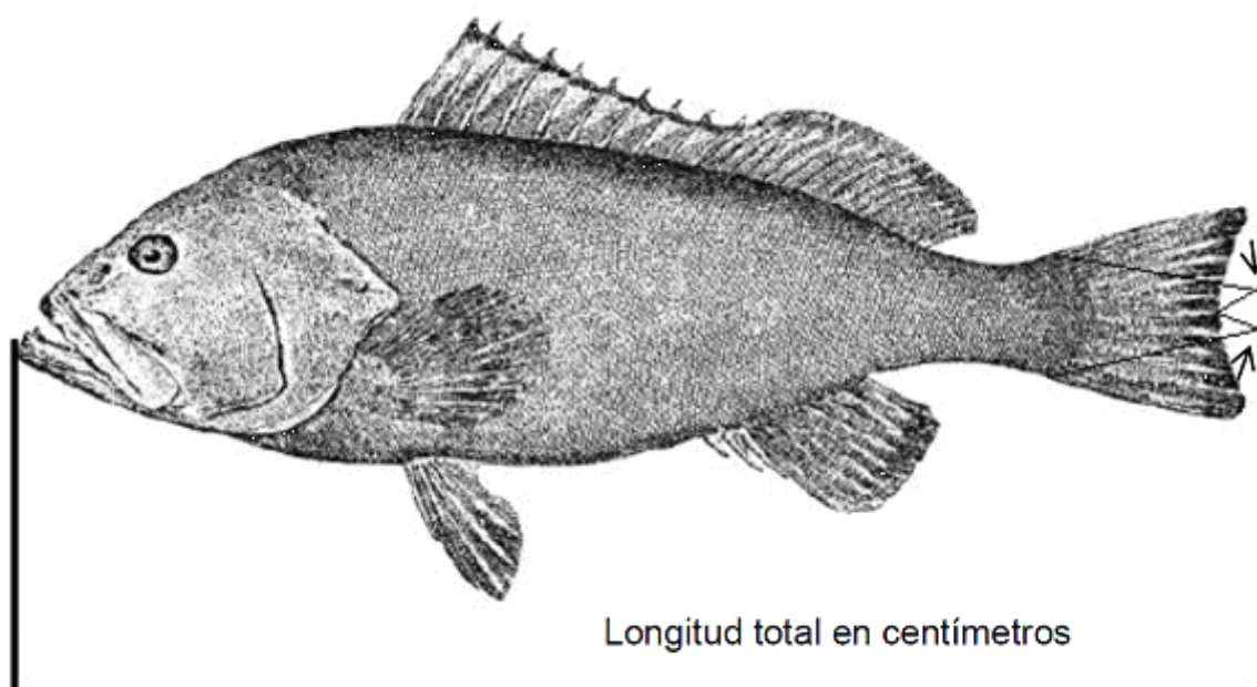
Fig. 1 Longitud total del mero rojo ( Epinephelus morio )
