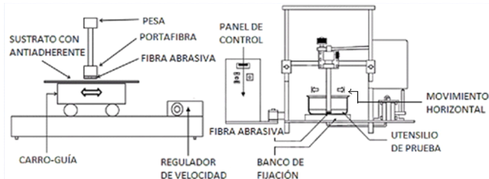
Figura 3 - Ejemplo de equipos para la prueba de abrasión o duración
