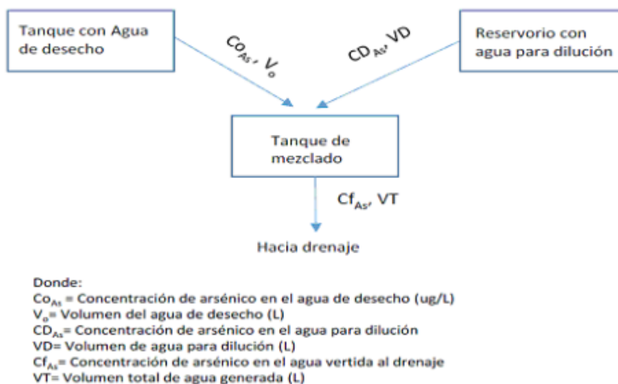
Figura G.3 Diagrama del balance de masa para la disolución de arsénico en el agua vertida a la red
