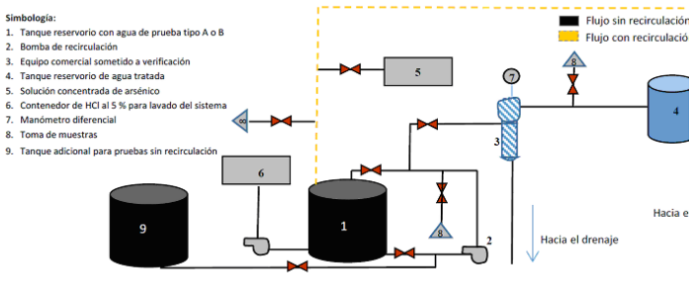
Figura G.1. Montaje para la verificación de equipos en la remoción de Arsénico en Agua para uso y consumo humano.
