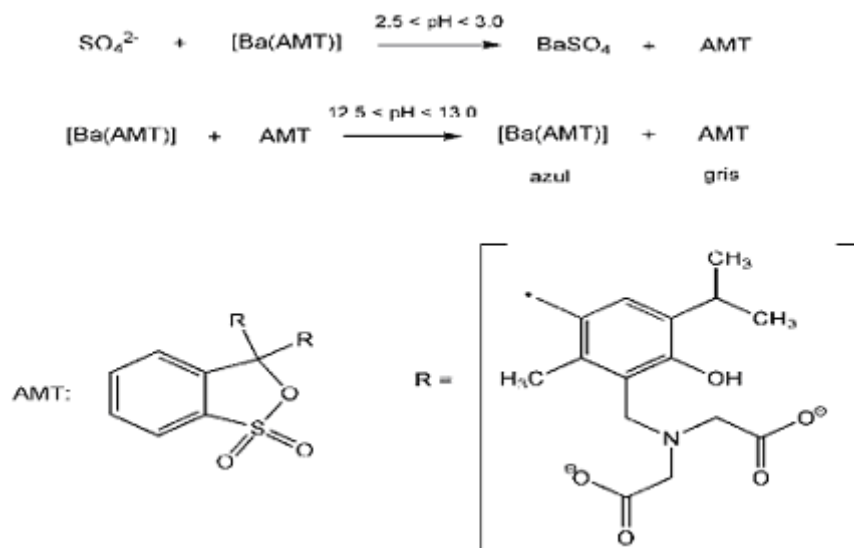
Fig. B.11.2-1. Reacción entre el Ion sulfato y el complejo bario azul de metiltímol (Ba-AMT).
